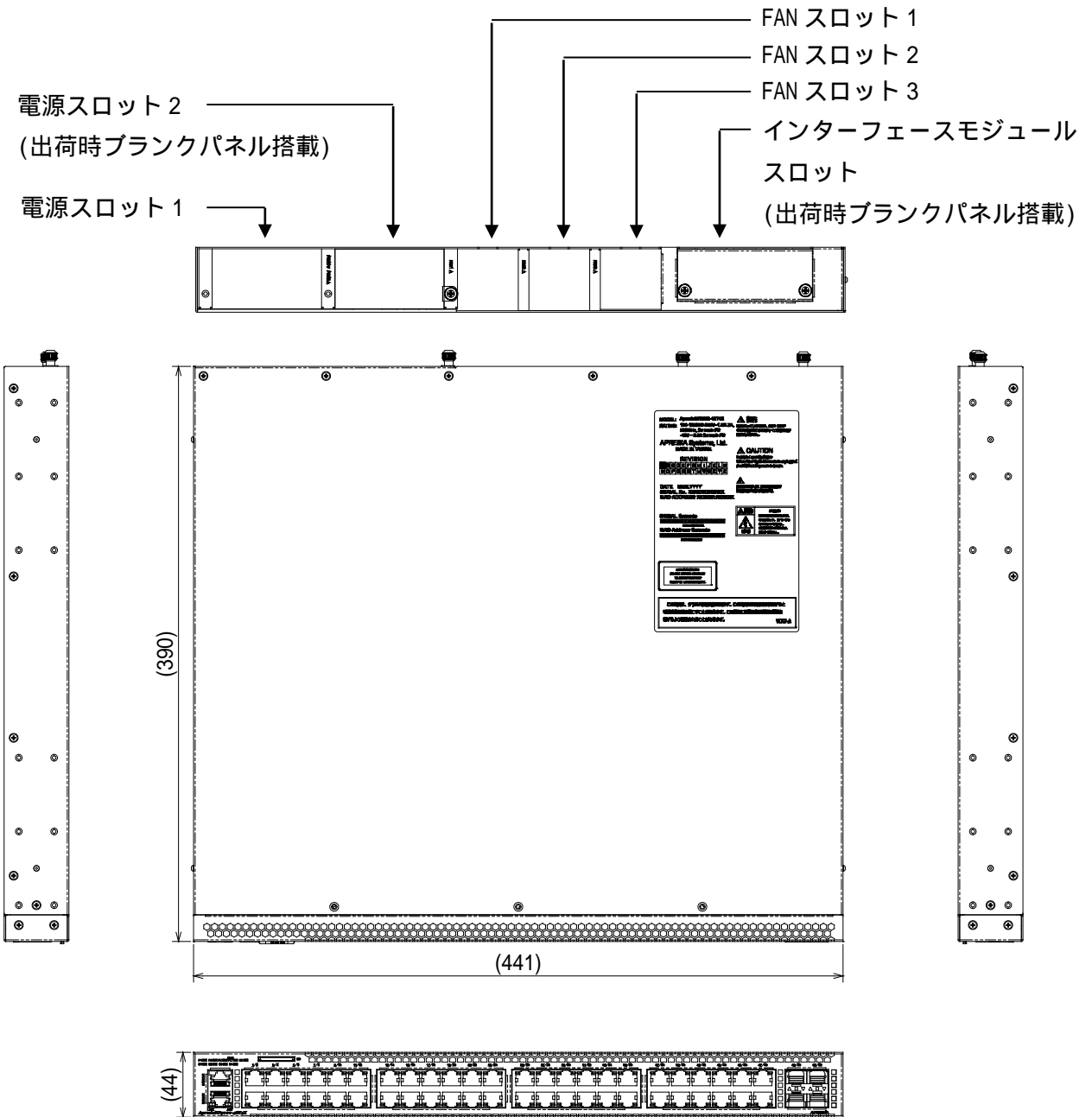
図 10-1 ApresiaNP5000-48T4X 外觀図 (Rev.A)
