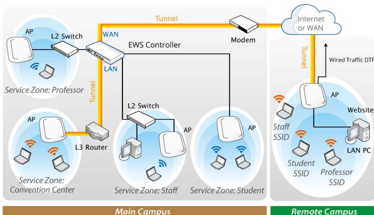
【レイヤ3 トポロジのグラフィック図】
