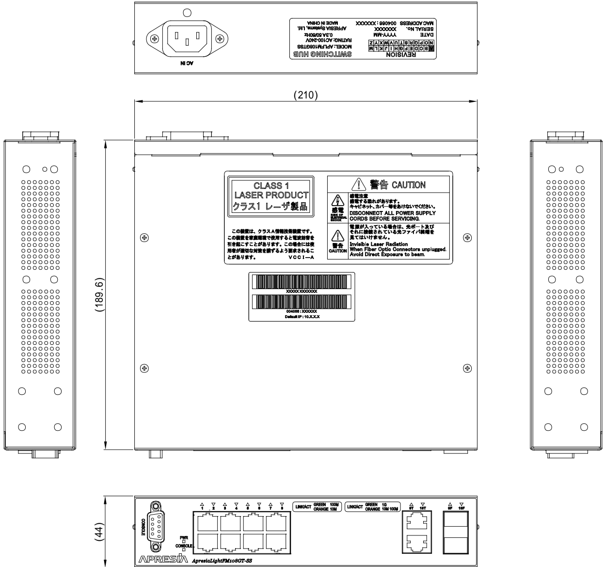
図 11-1 ApresiaLightFM108GT-SS 外観図
