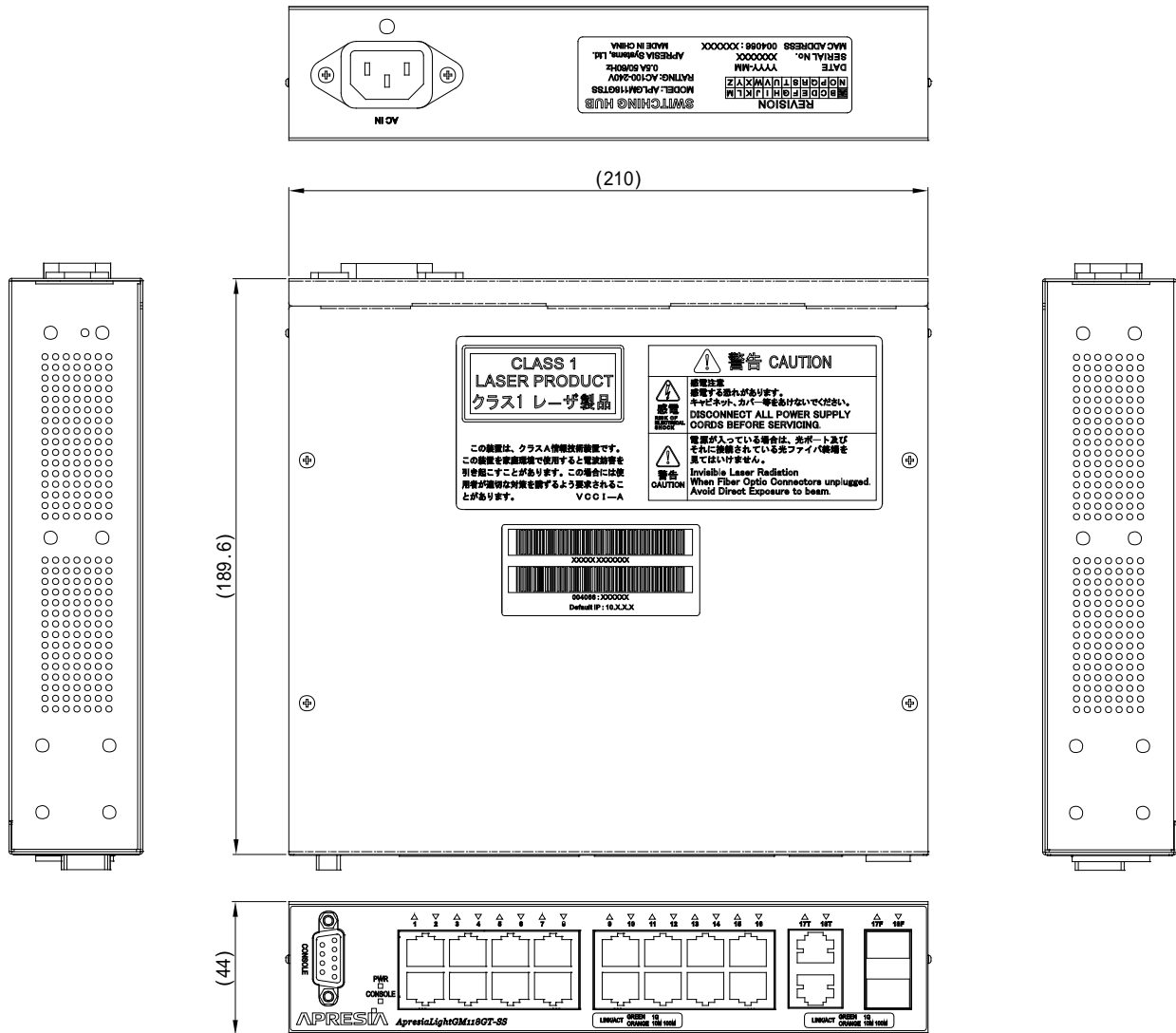
図 11-1 ApresiaLightGM118GT-SS 外観図
