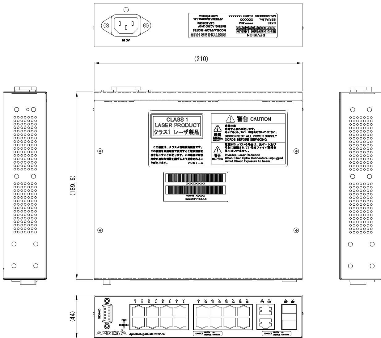
図 11-1 ApresiaLightGM118GT-SS 外観図
