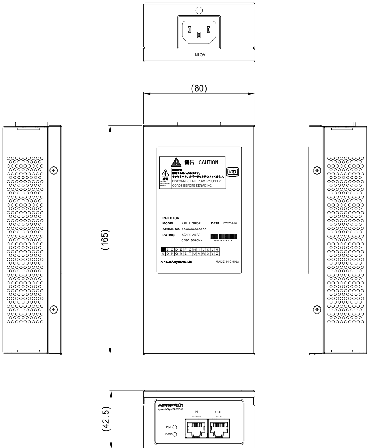
図 10-1 ApresiaLightIJ-1GPoE 外観図
