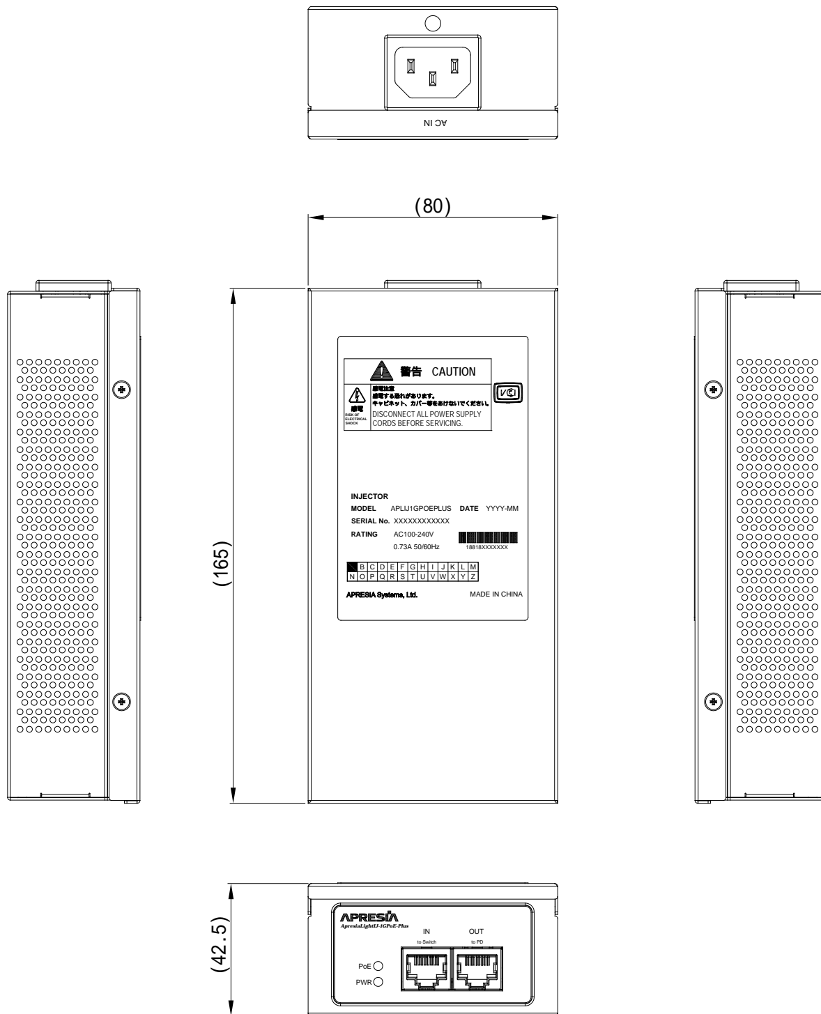
図 10-2 ApresiaLight IJ-1GPoE-Plus 外観図
