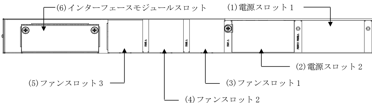
図 2-7 ApresiaNP5000-48T4X のリアパネル
