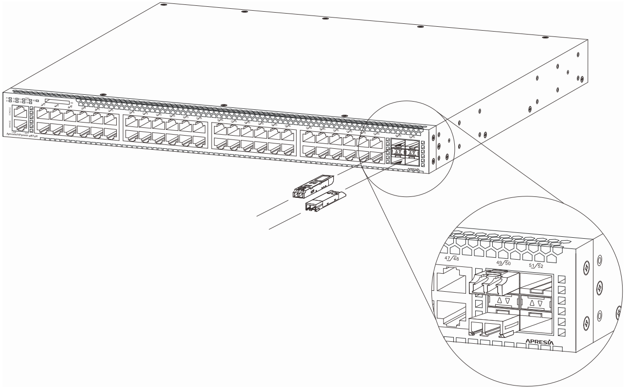
図 3-9 ApresiaNP5000-48T4X、ApresiaNP4000-20Xt4X、ApresiaNP2000-48T4X SFP、SFP+挿入向き
