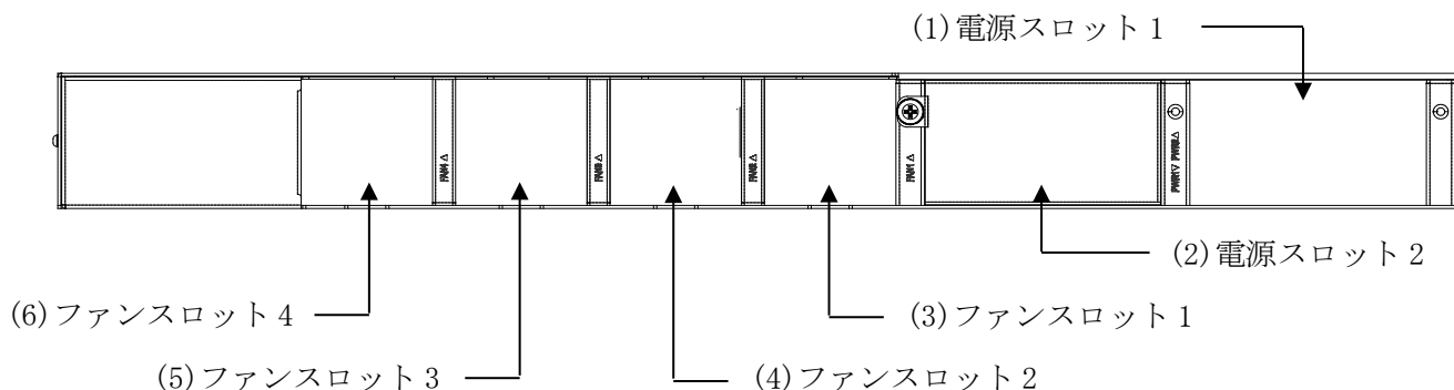
図 2-6 ApresiaNP7000-48X6L のリアパネル
