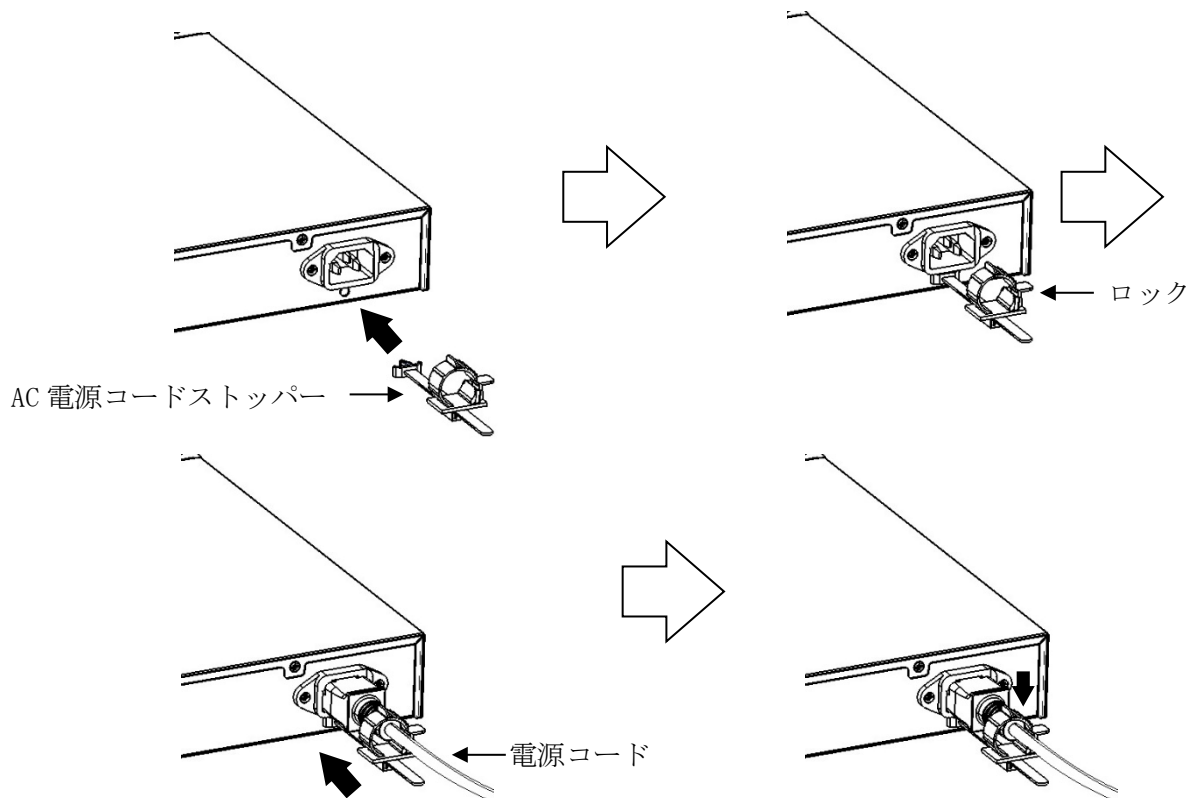
図 3-16 AC 電源コード、AC 電源コードストッパーの接続 (ApresiaNP4000-20Xt4X、ApresiaNP2000-24T4X、ApresiaNP2000-48T4X)
