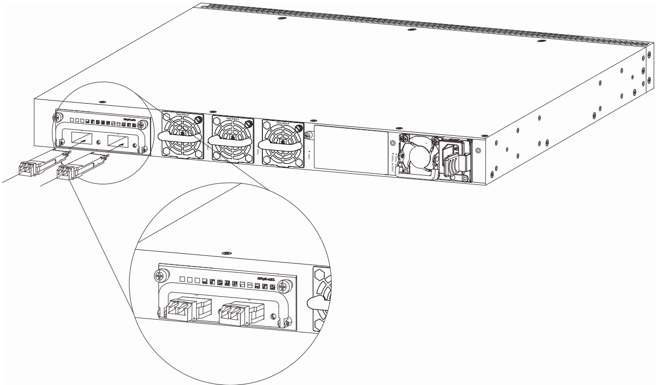
図 3-10 ApresiaNP5000-48T4X QSFP+挿入向き
