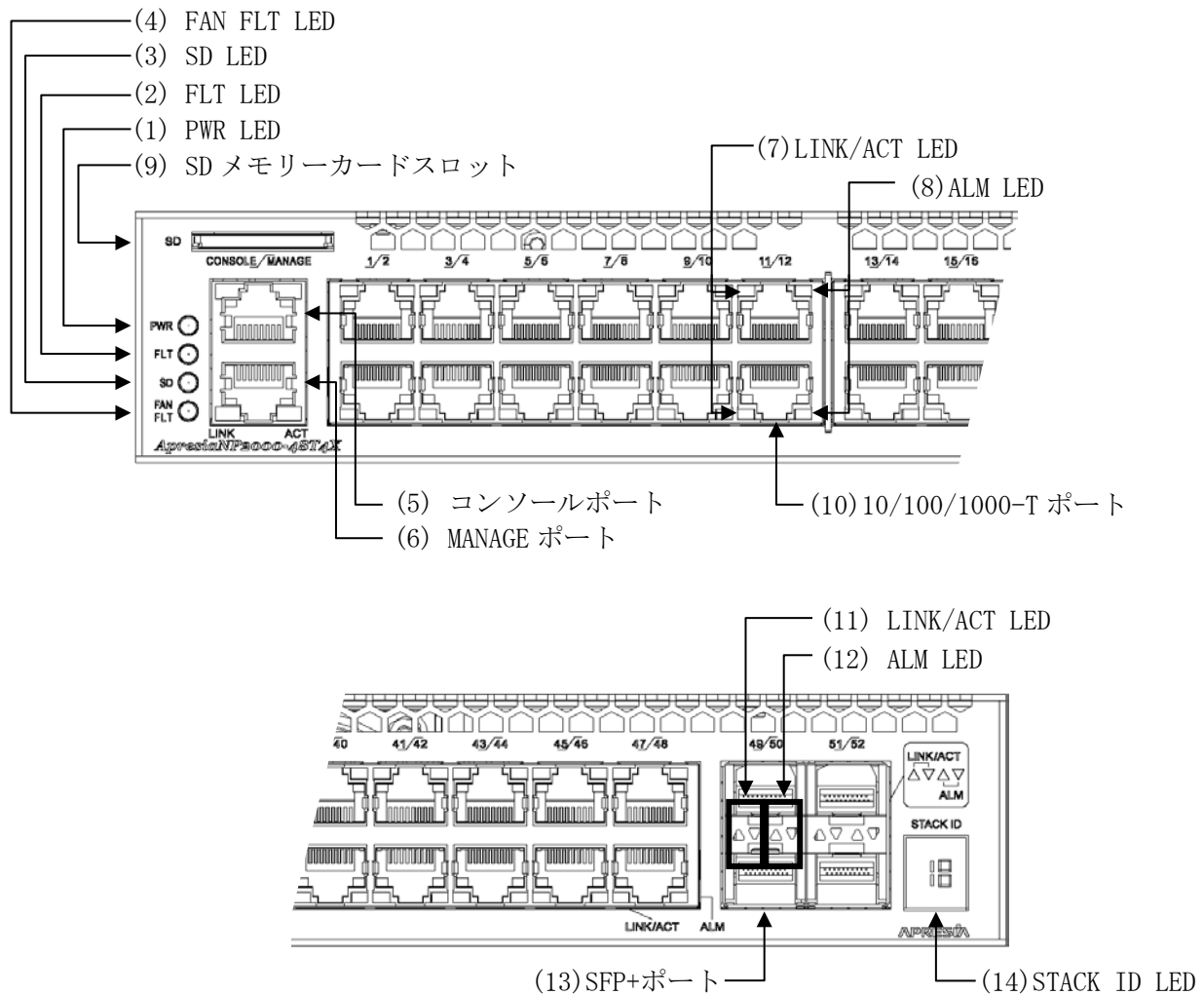
図 2-5 ApresiaNP2000-48T4X フロントパネルの構成
