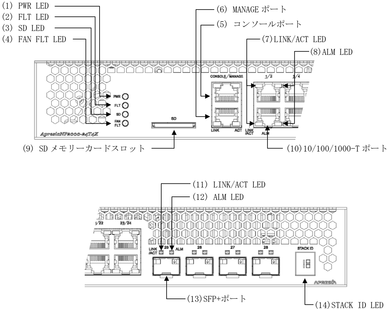
図 2-4 ApresiaNP2000-24T4X フロントパネルの構成
