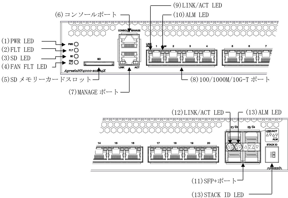
図 2-3 ApresiaNP4000-20Xt4X フロントパネルの構成
