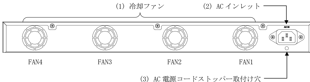
図 2-8 ApresiaNP4000-20Xt4X のリアパネル
