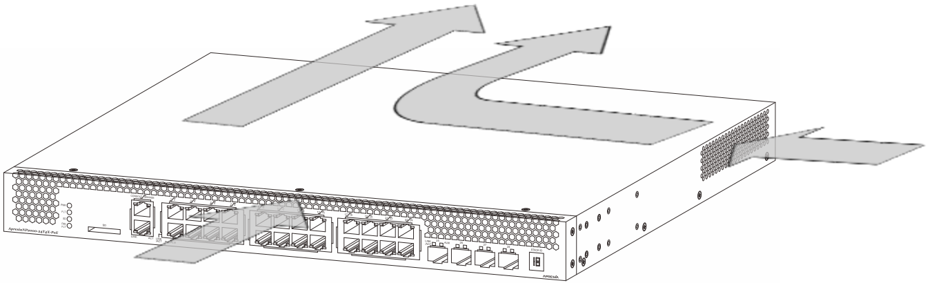
图 3-5 ApresiaNP2000-24T4X-PoE、ApresiaNP2000-48T4X-PoE
