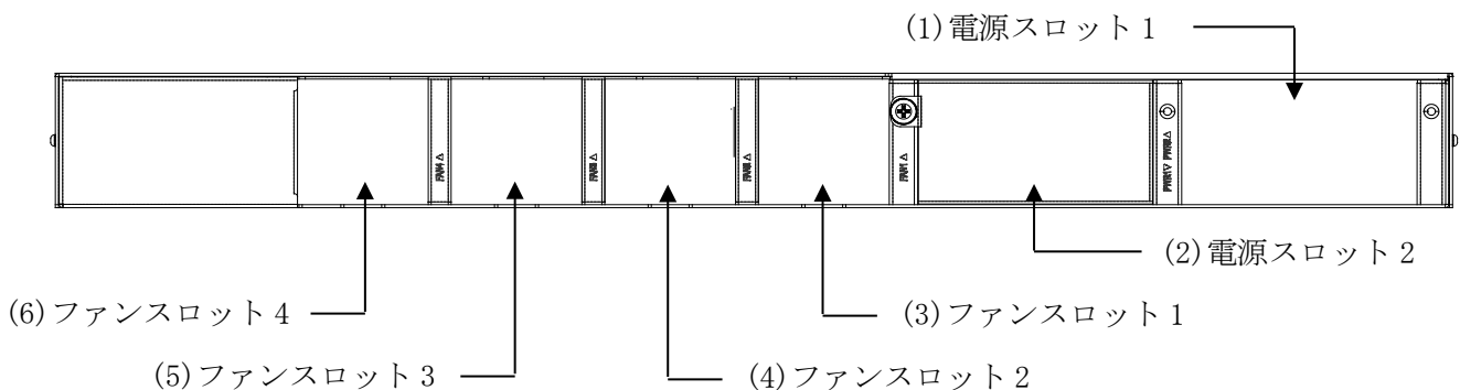
図 2-15 ApresiaNP7000-48X6L、ApresiaNP7000-24G24X6L のリアパネル
