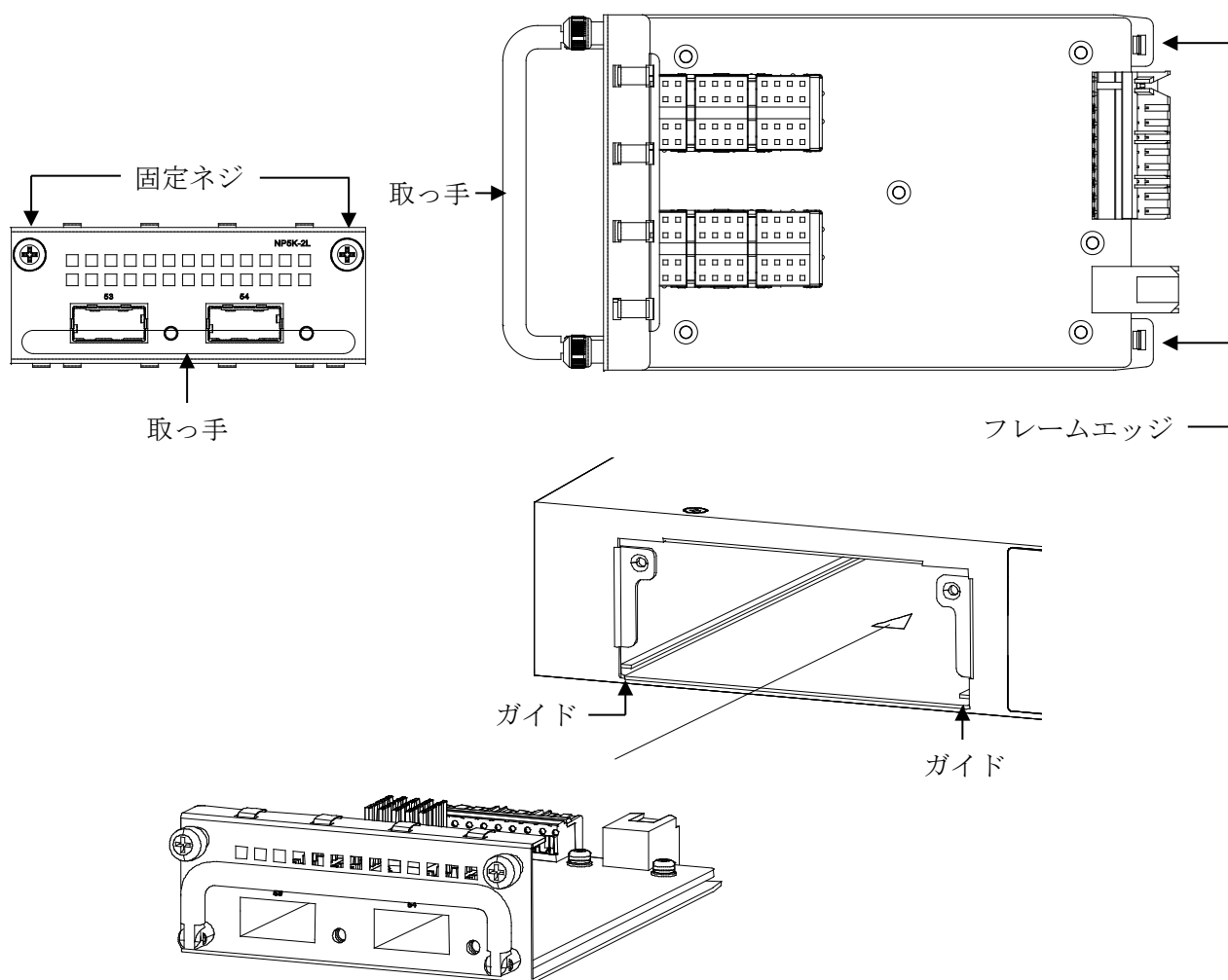
図 3-15 インターフェースモジュールの装着方法
