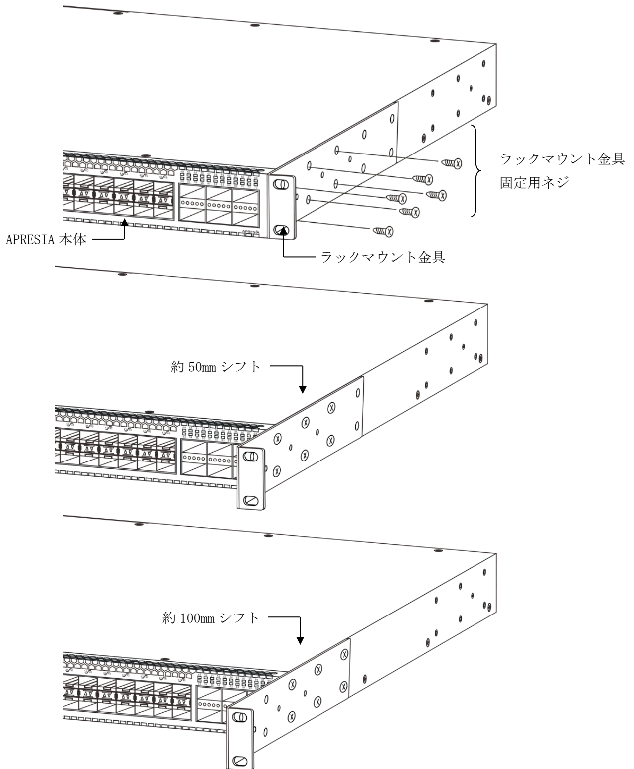
図 3-7 標準添付 0mm、50mm、100mm シフトラックマウント金具の取り付け方法
