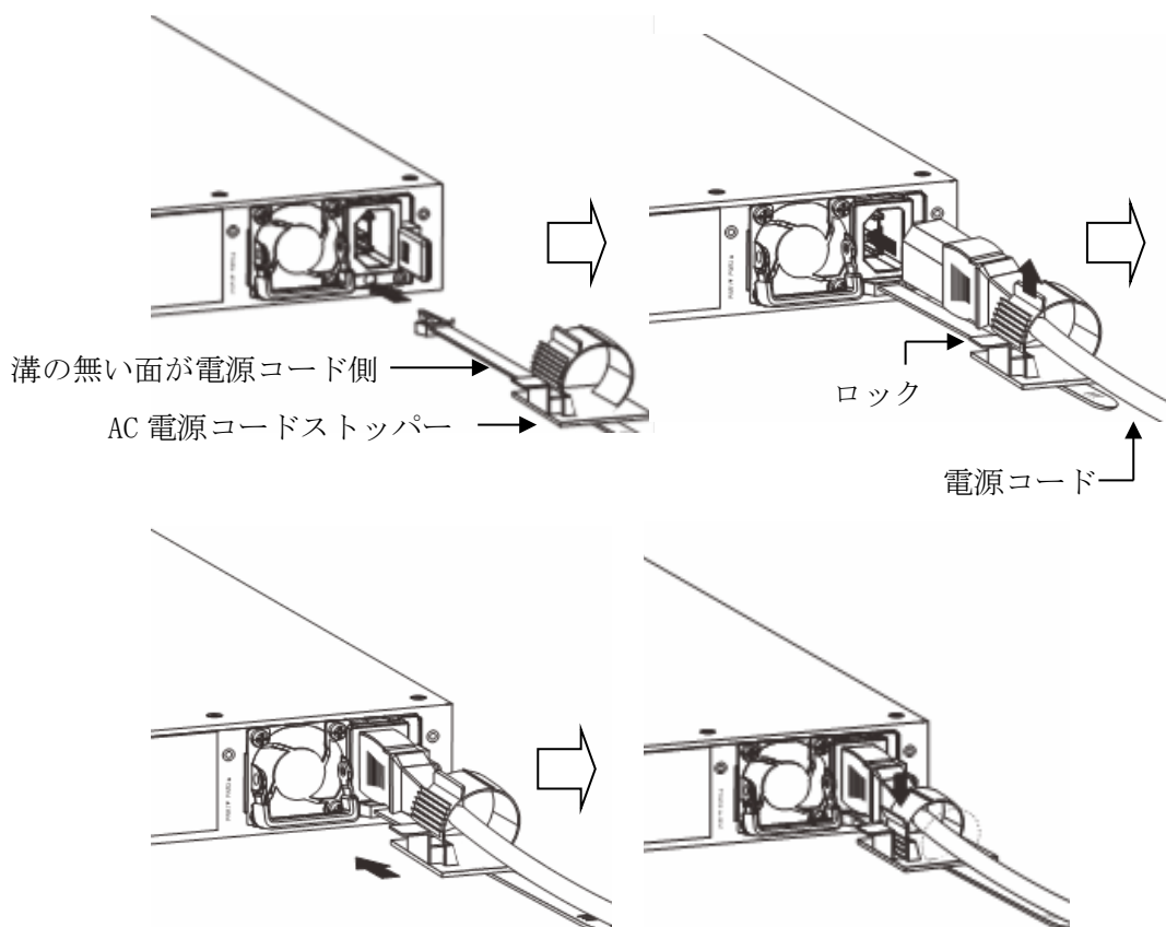
図 3-26 AC 電源コード、AC 電源コードストッパーの接続 (ApresiaNP7000-48X6L、ApresiaNP7000-24G24X6L、ApresiaNP5000-48T4X)
