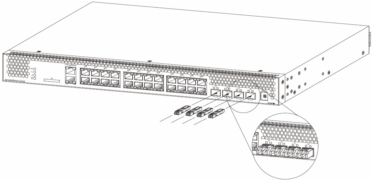
図 3-20 ApresiaNP2100-24T4X、ApresiaNP2100-24T4X-PoE、ApresiaNP2000-24T4X、ApresiaNP2000-24T4X-PoE SFP、SFP+挿入向き
