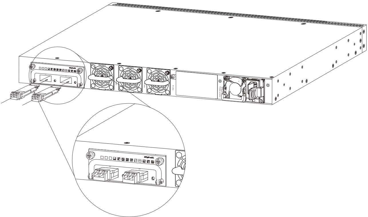
図 3-19 ApresiaNP5000-48T4X QSFP+挿入向き
