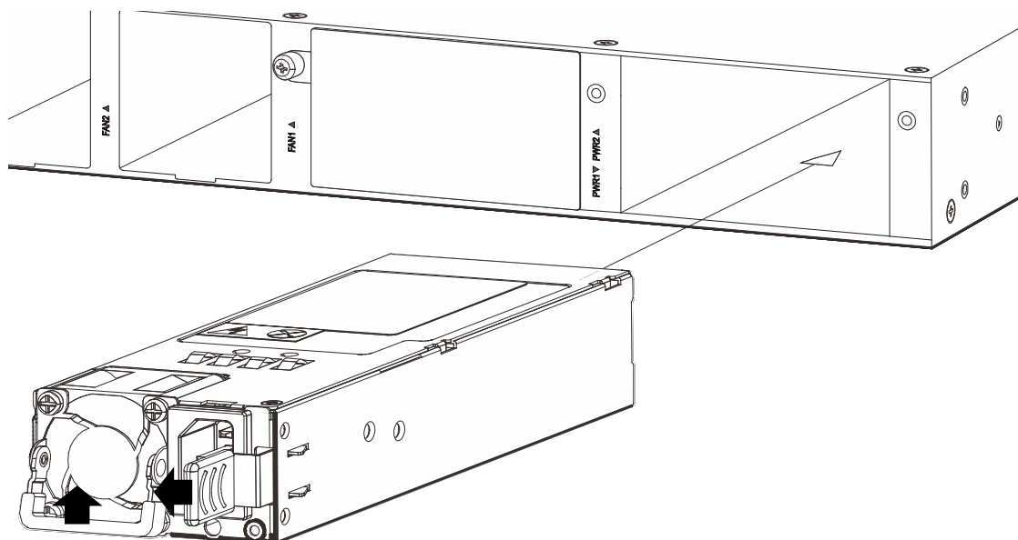
図 3-24 電源ユニットの装着方法
