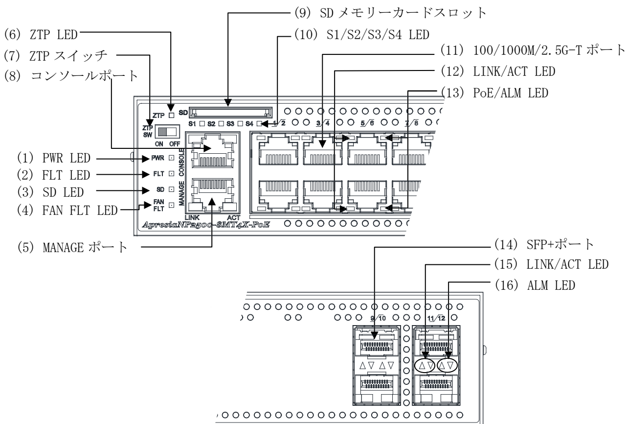
図 2-5 ApresiaNP2500-8MT4X-PoE フロントパネルの構成
