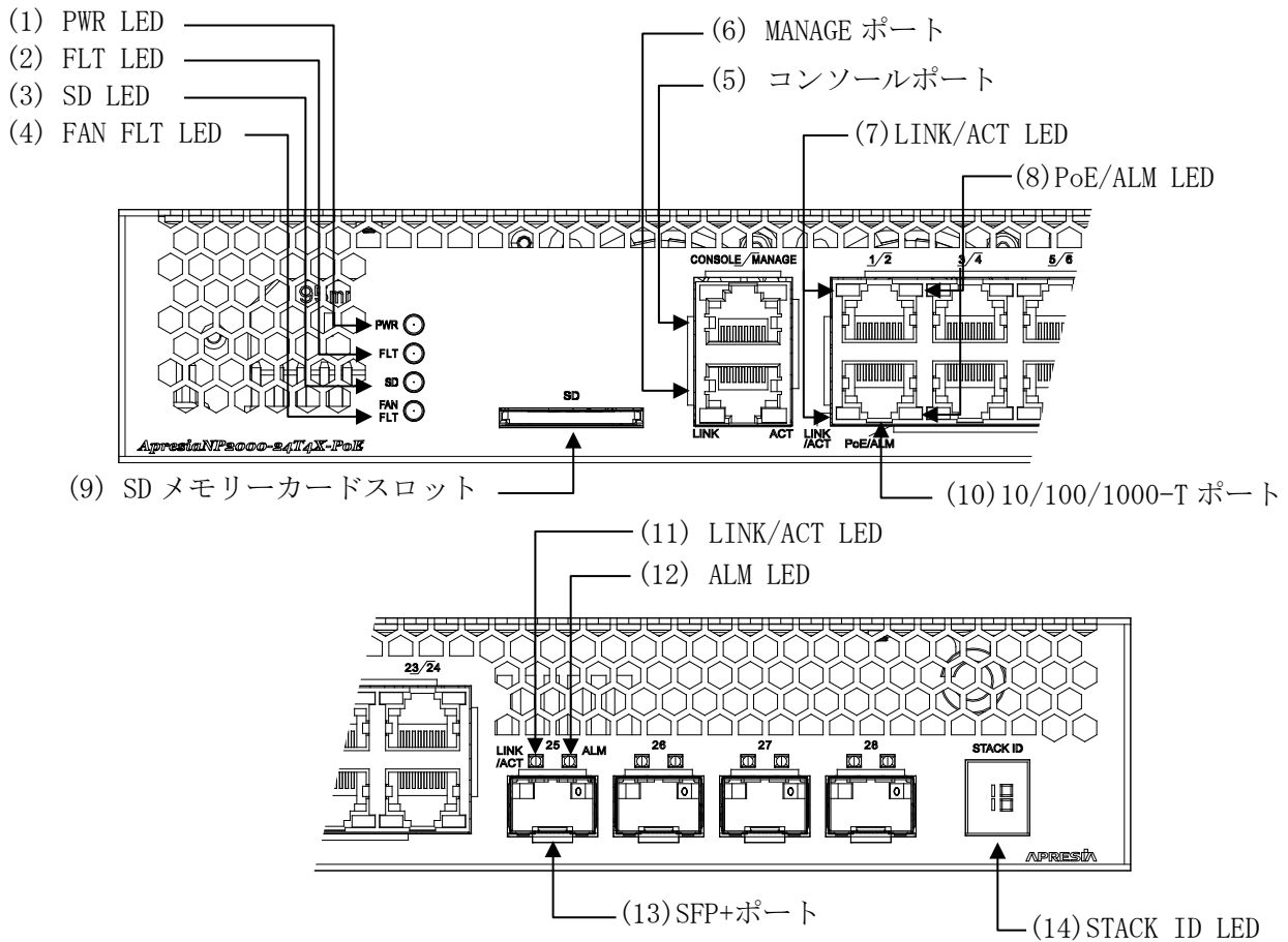
図 2-12 ApresiaNP2000-24T4X-PoE フロントパネルの構成
