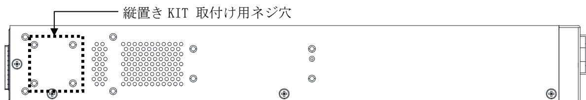
図 3-11 ApresiaNP2500-8MT4X-PoE、ApresiaNP2500-48T4X-PoE 縦置き KIT 取り付けネジ穴位置
