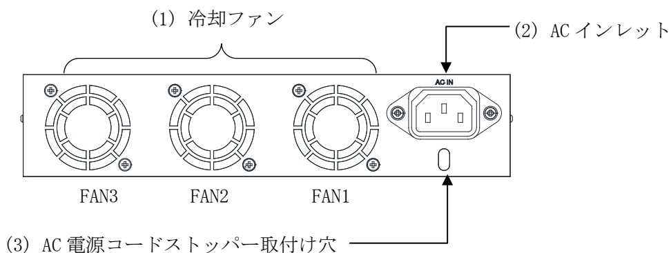
図 2-18 ApresiaNP2500-8MT4X-PoE、ApresiaNP2500-16MT4X-PoE のリアパネル
