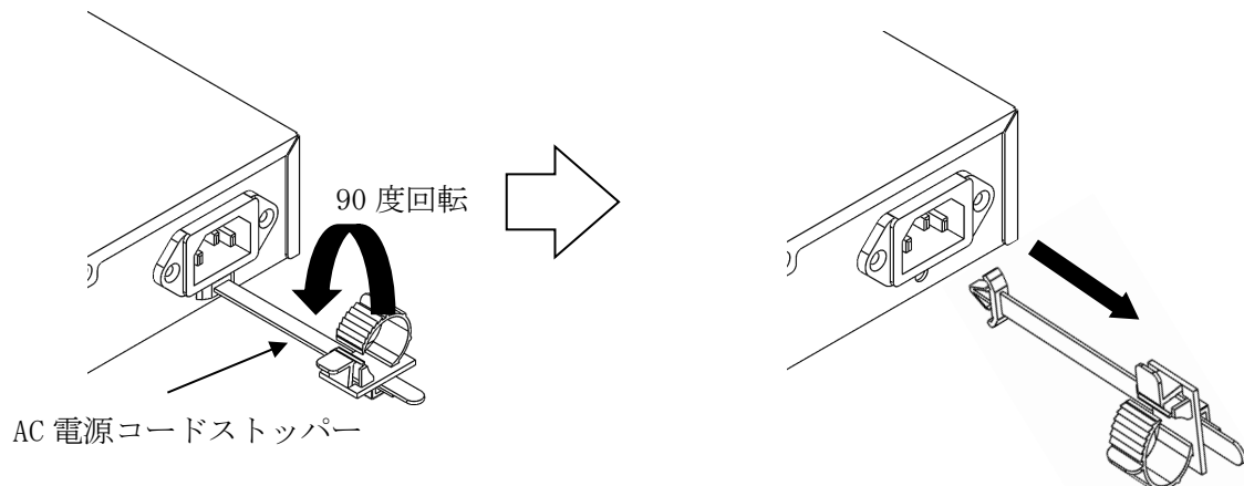
図 3-28 AC 電源コードの抜き取り
