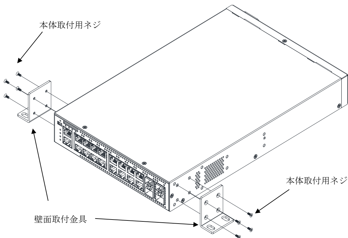
図 3-14 壁面取付金具(AL-WM)の取り付け方法
