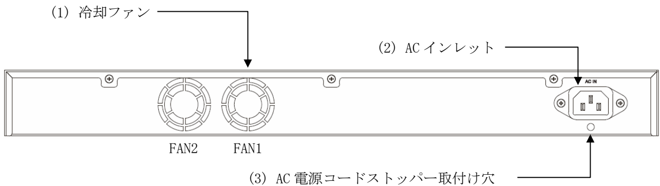
図 2-19 ApresiaNP2100-24T4X、ApresiaNP2100-48T4X、ApresiaNP2000-24T4X、ApresiaNP2000-48T4X のリアパネル
