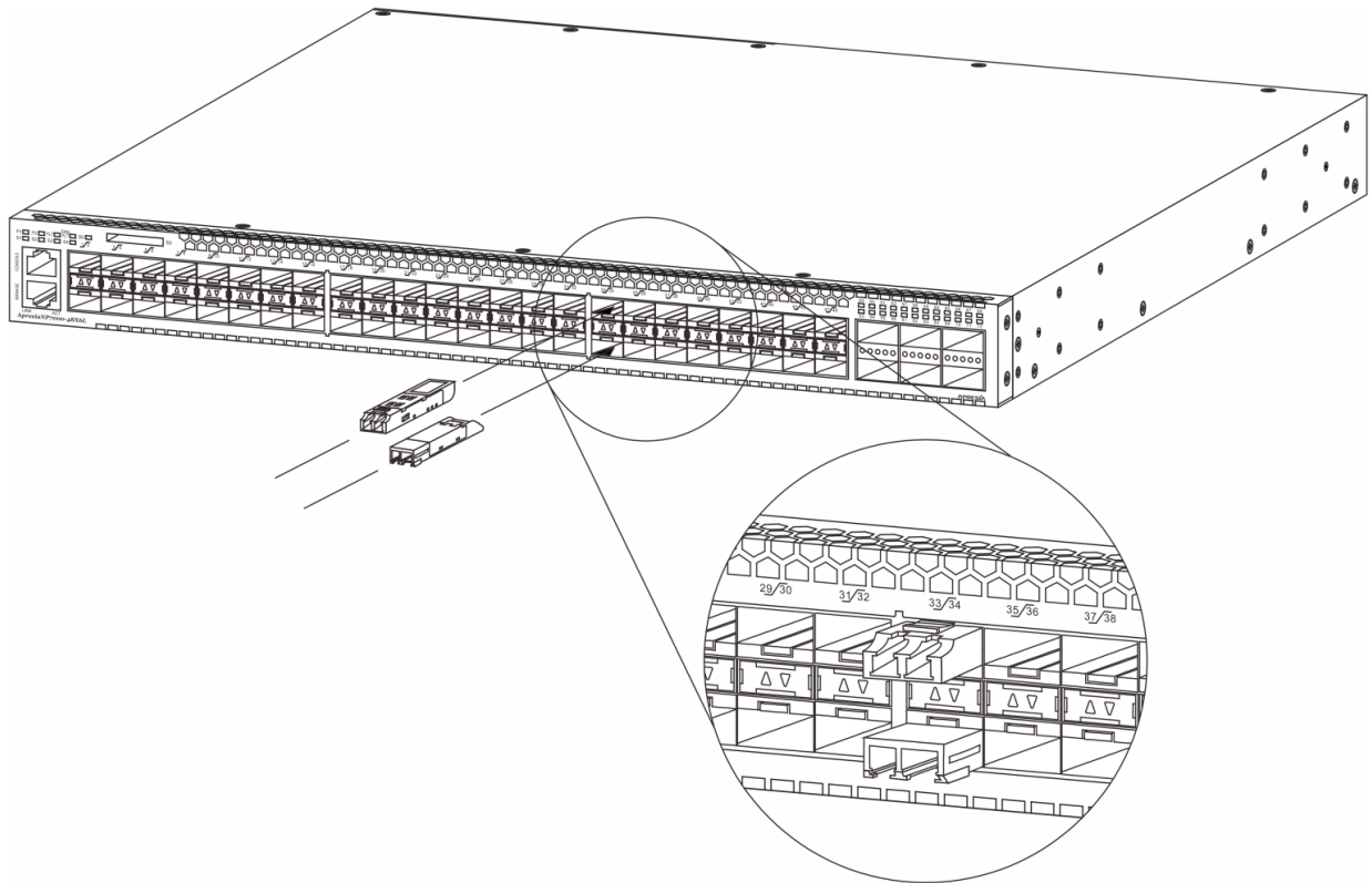
図 3-16 ApresiaNP7000-48X6L、ApresiaNP7000-24G24X6L SFP、SFP+挿入向き
