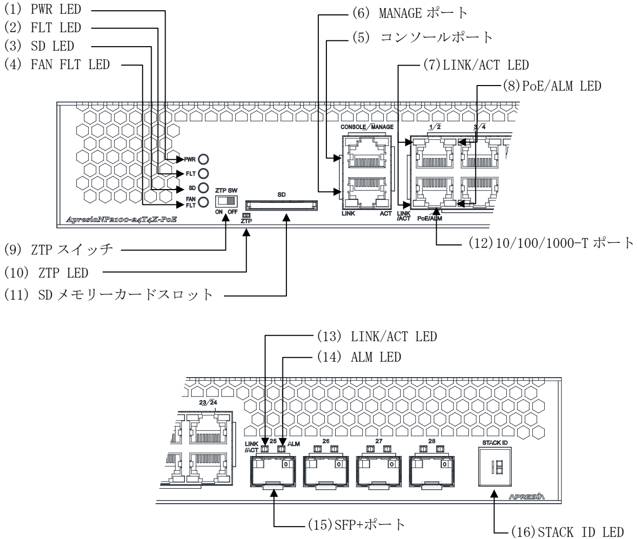
図 2-8 ApresiaNP2100-24T4X-PoE フロントパネルの構成
