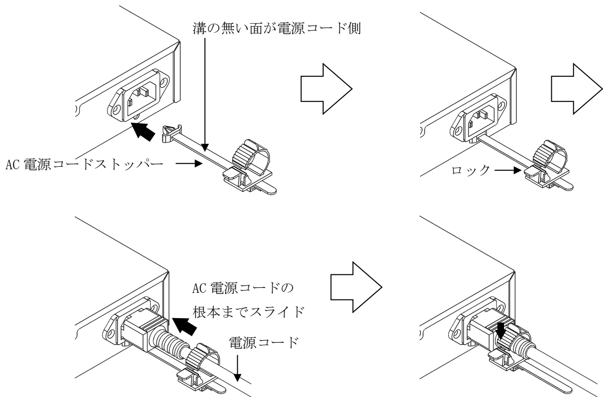
図 3-27 AC 電源コード、AC 電源コードストッパーの接続
