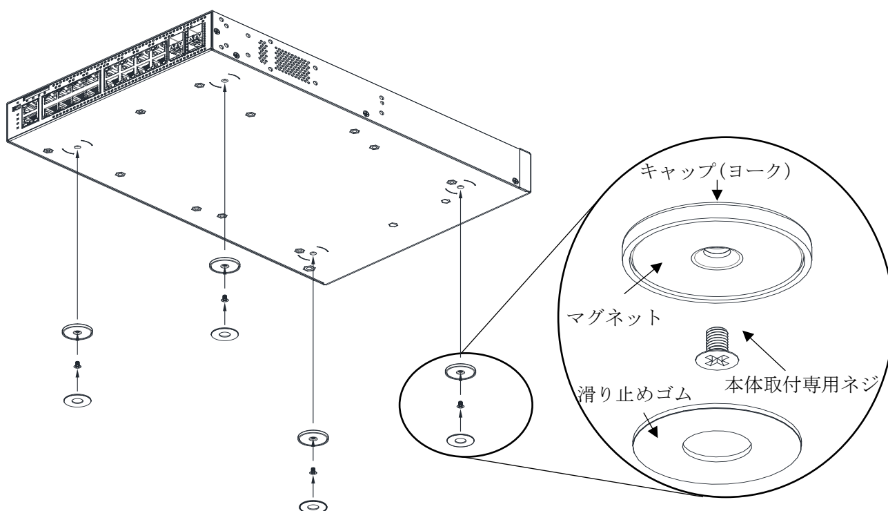
図 3-13 マグネット(AL-MG-B04)の取り付け方法
