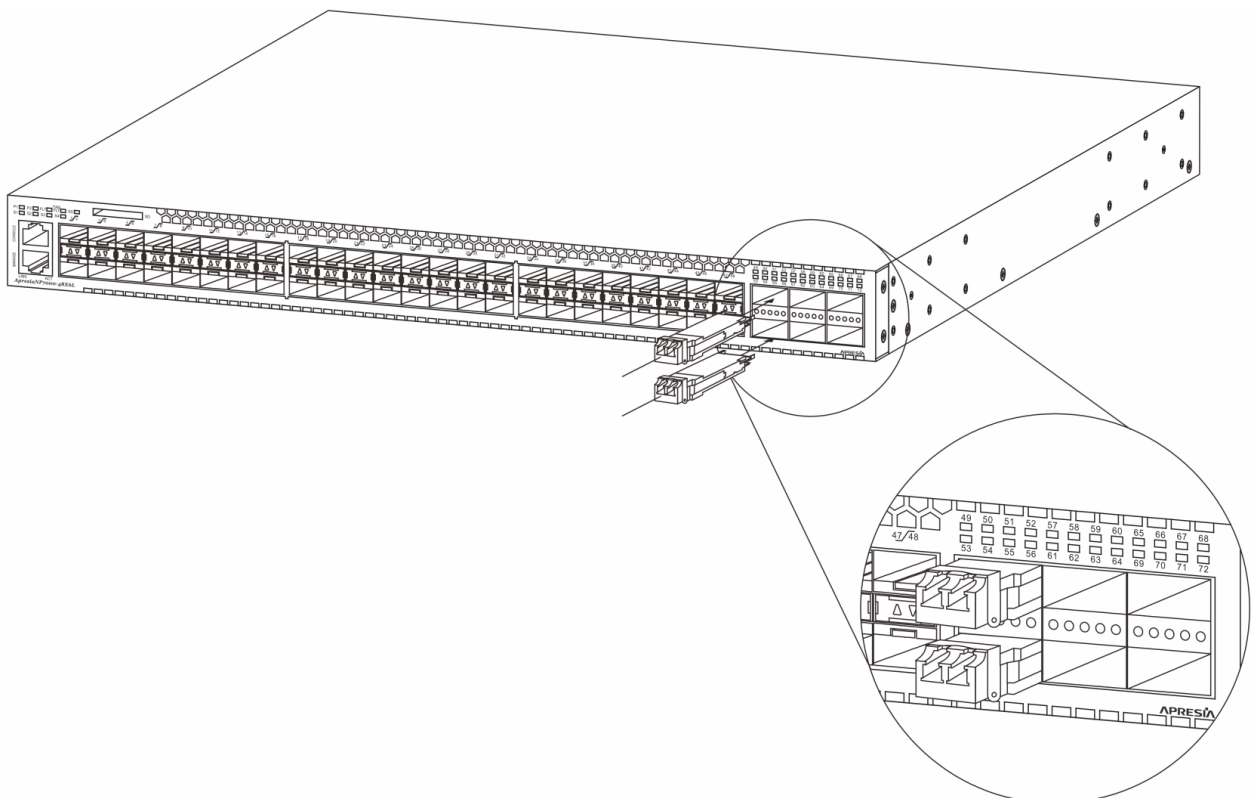
図 3-17 ApresiaNP7000-48X6L、ApresiaNP7000-24G24X6L QSFP+挿入向き
