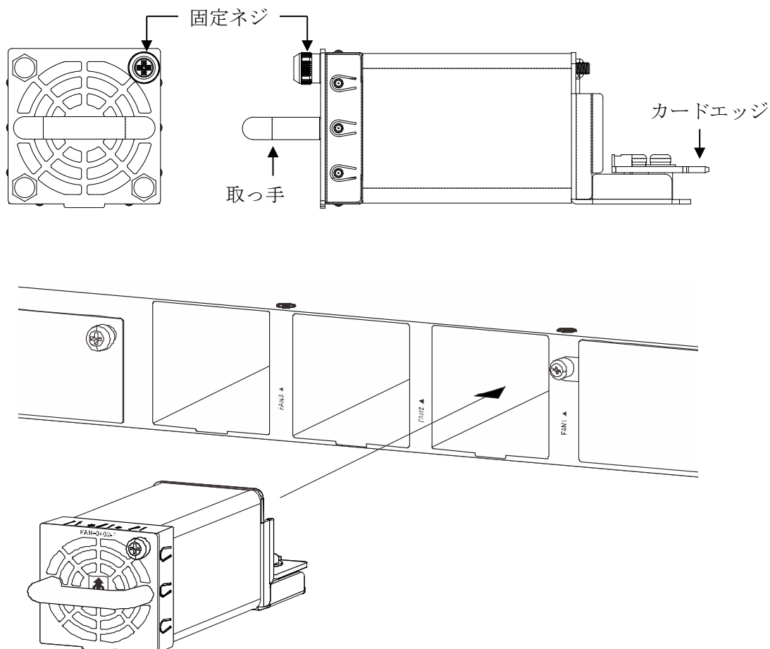
図 3-23 ファンユニットの装着方法
