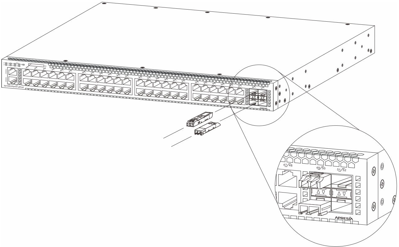
図 3-18 ApresiaNP5000-48T4X、ApresiaNP4000-20Xt4X、ApresiaNP2500-8MT4X-PoE、ApresiaNP2500-16MT4X-PoE、ApresiaNP2100-48T4X、ApresiaNP2100-48T4X-PoE、ApresiaNP2000-48T4X、ApresiaNP2000-48T4X-PoE SFP、SFP+挿入向き
