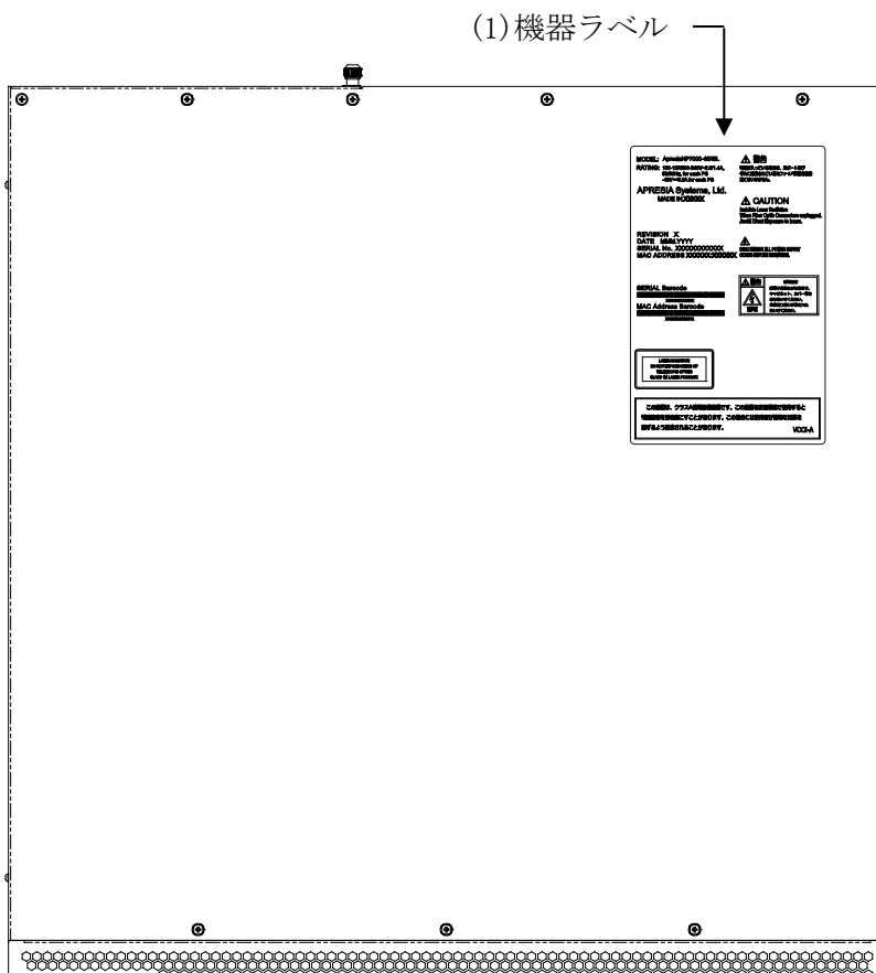
図 2-21 ApresiaNP7000-48X6L のトップパネル
