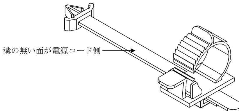
図 3-25 AC 電源コードストッパーの組立て方
