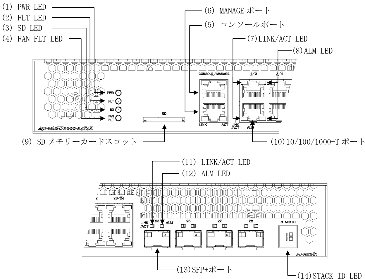
図 2-11 ApresiaNP2000-24T4X フロントパネルの構成
