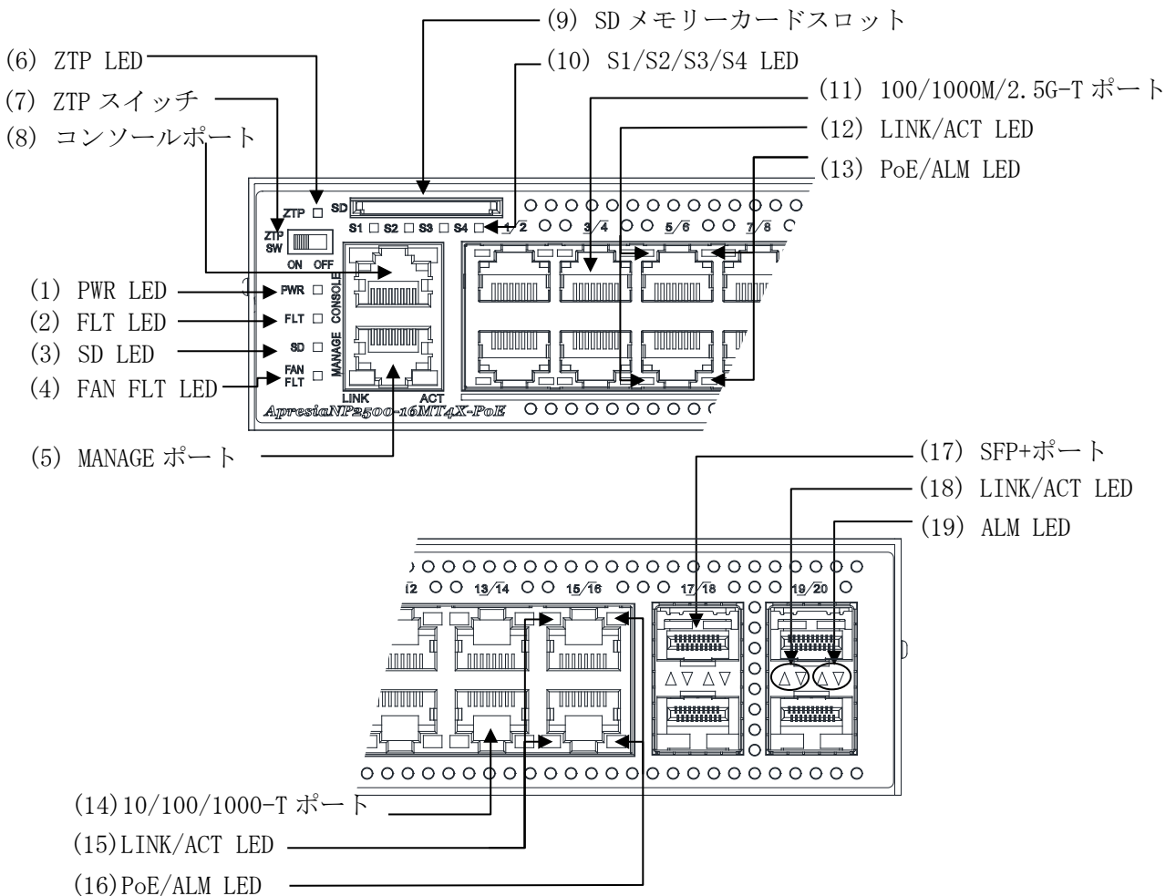
図 2-6 ApresiaNP2500-16MT4X-PoE フロントパネルの構成
