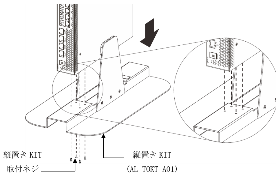
図 3-10 縦置き KIT (AL-TOKT-A01) の取り付け方法
