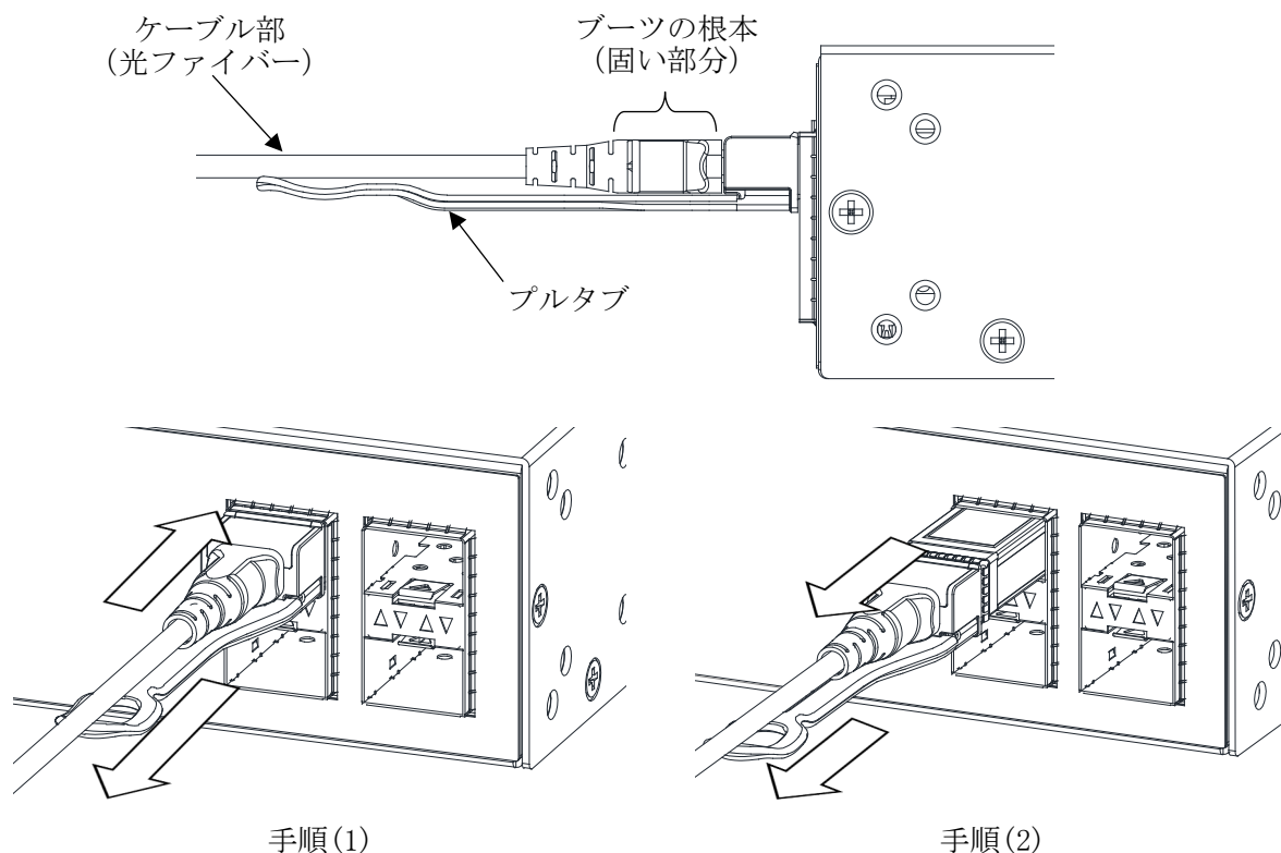
図 3-21 SFP+ AOC の取り外し方法 (製品型式 H-SFP+AOCxM の例)
