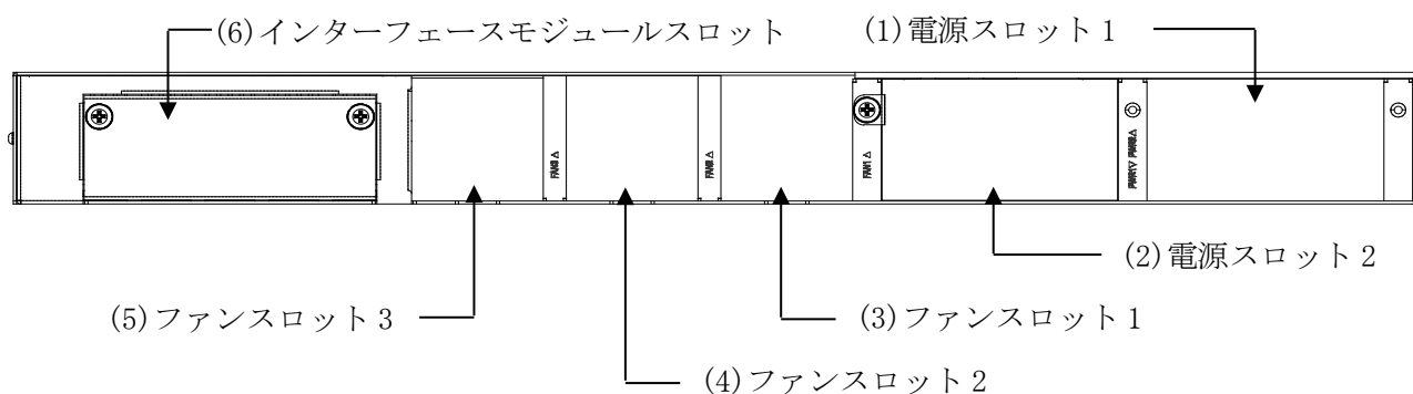
図 2-16 ApresiaNP5000-48T4X のリアパネル
