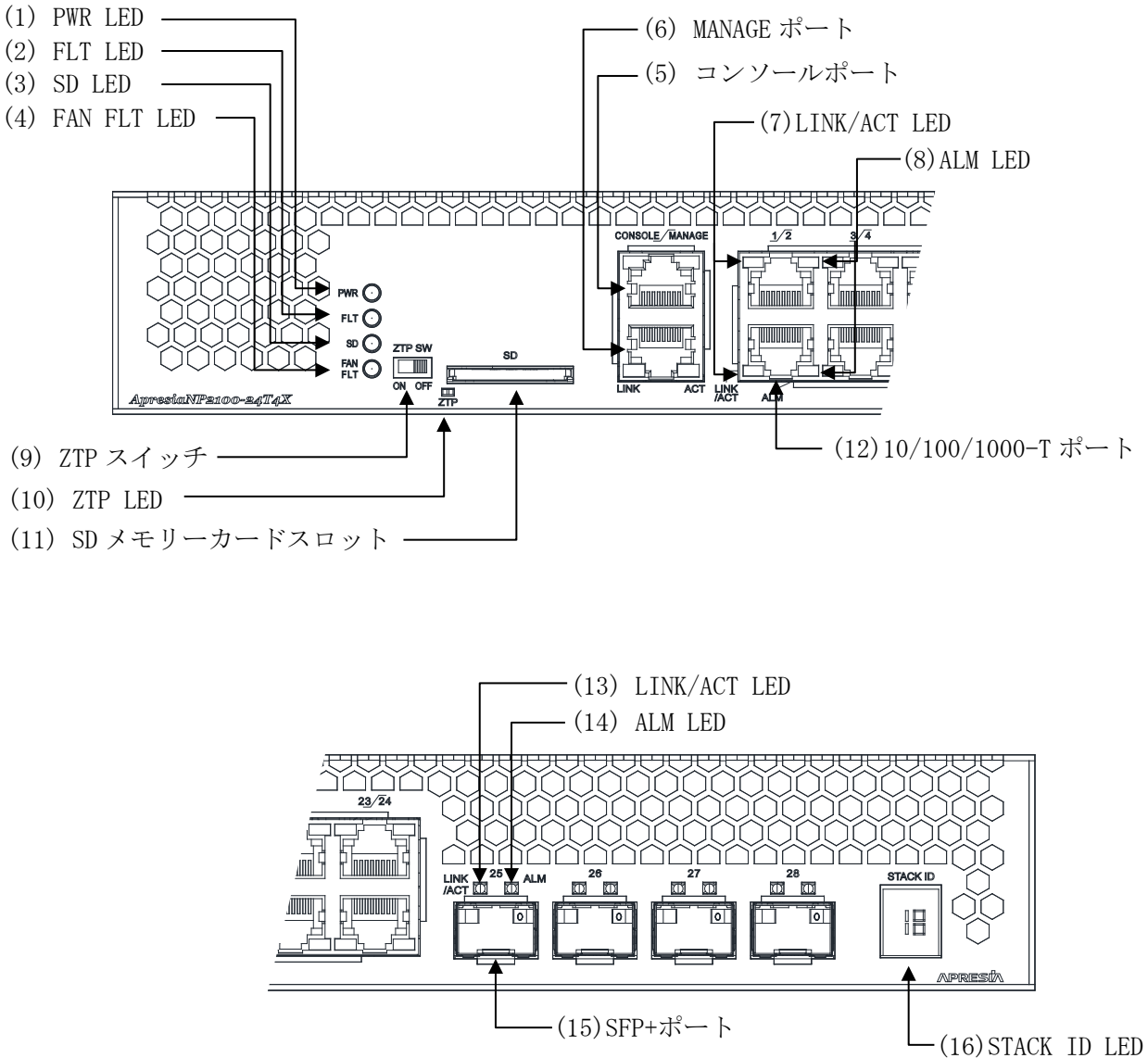
図 2-7 ApresiaNP2100-24T4X フロントパネルの構成
