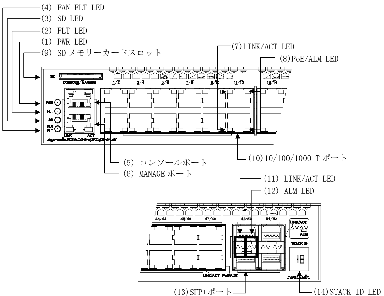
図 2-14 ApresiaNP2000-48T4X-PoE フロントパネルの構成
