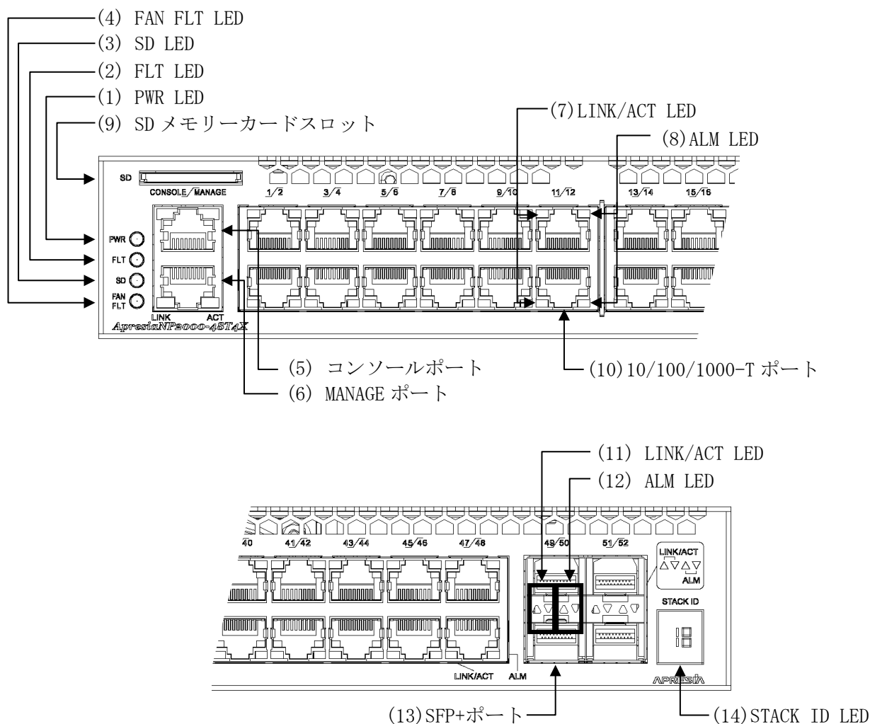
図 2-13 ApresiaNP2000-48T4X フロントパネルの構成
