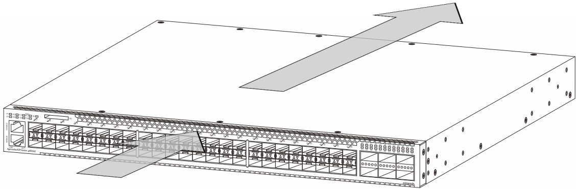
図 3-3 ApresiaNP7000-48X6L(前面吸気背面排気)、ApresiaNP7000-24G24X6L(前面吸気背面排気)、 ApresiaNP5000-48T4X(前面吸気背面排気)、ApresiaNP4000-20Xt4X、ApresiaNP2100-24T4X、 ApresiaNP2100-48T4X、ApresiaNP2000-24T4X、ApresiaNP2000-48T4X
