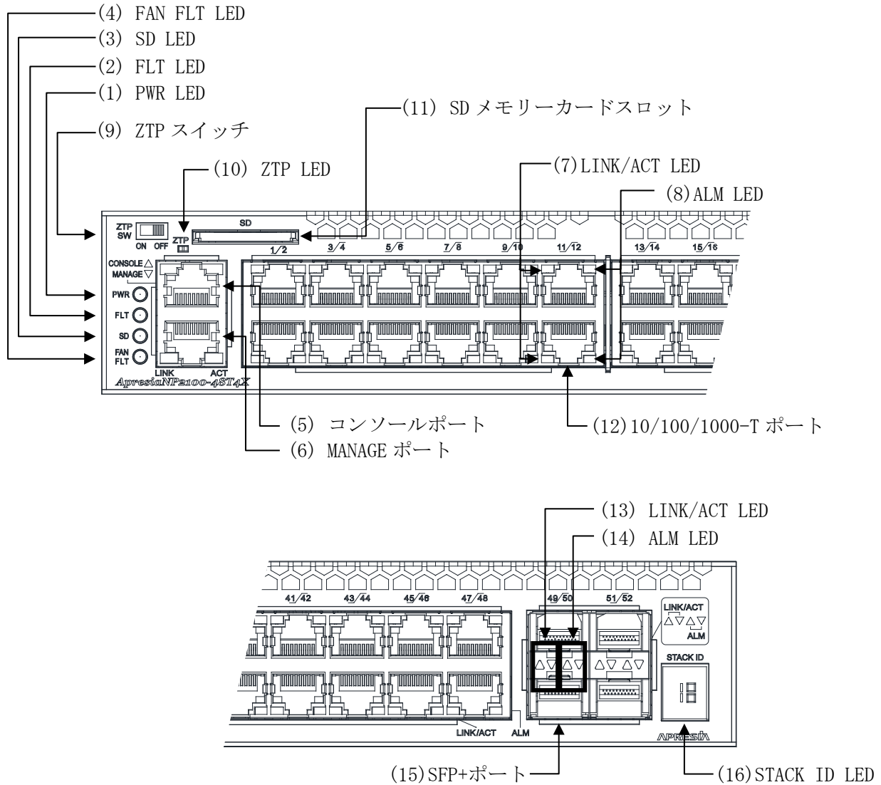
図 2-9 ApresiaNP2100-48T4X フロントパネルの構成
