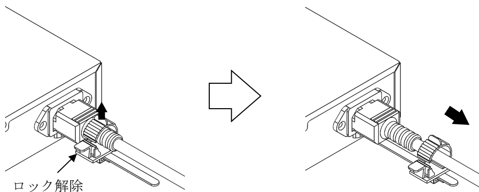
図 3-28 AC 電源コードの抜き取り
