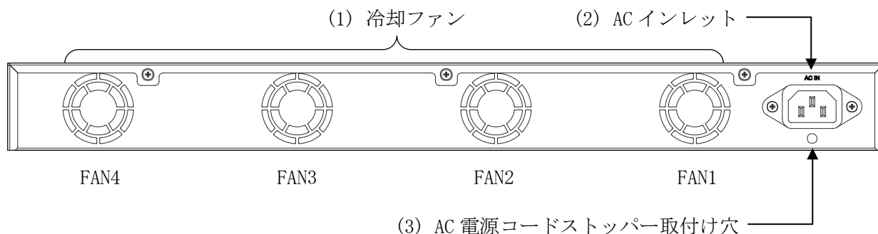
図 2-17 ApresiaNP4000-20Xt4X のリアパネル
