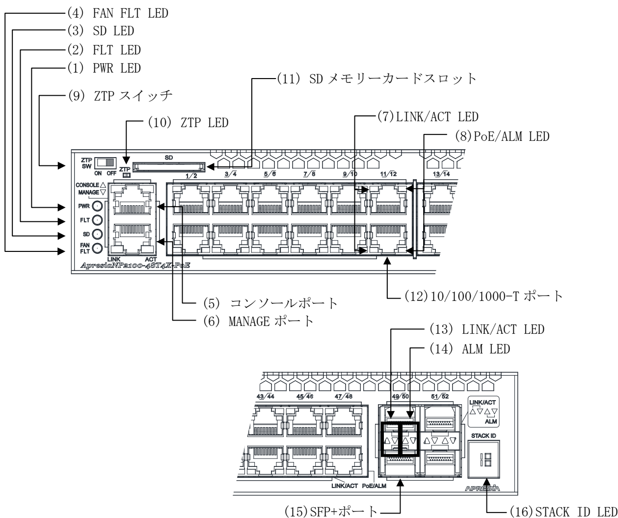
図 2-10 ApresiaNP2100-48T4X-PoE フロントパネルの構成
