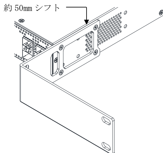
図 3-8 標準添付 0mm、50mm シフトラックマウント金具の取り付け方法
