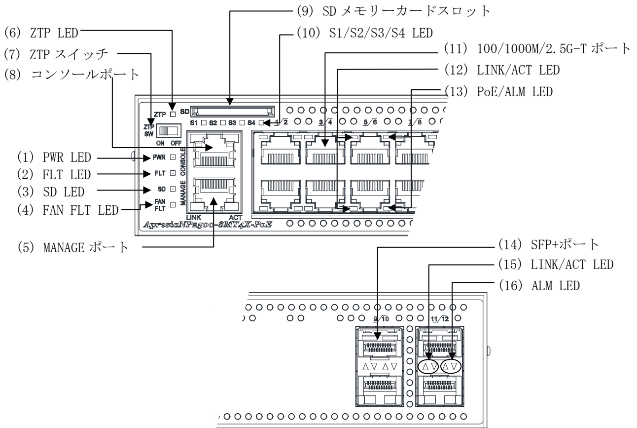
図 2-6 ApresiaNP2500-8MT4X-PoE フロントパネルの構成
