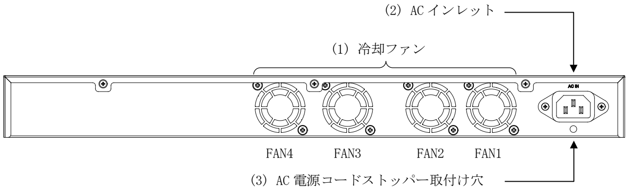
図 2-22 ApresiaNP2100-24T4X-PoE、ApresiaNP2100-48T4X-PoE、ApresiaNP2000-24T4X-PoE、ApresiaNP2000-48T4X-PoE のリアパネル
