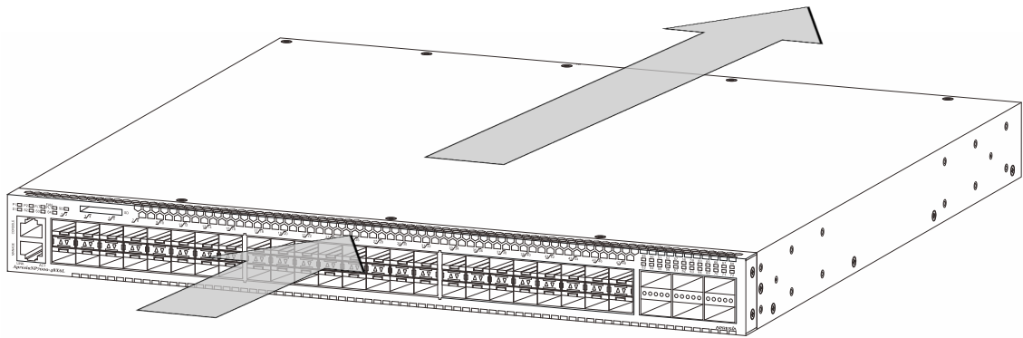
図 3-3 ApresiaNP7000-48X6L(前面吸気背面排気)、ApresiaNP7000-24G24X6L(前面吸気背面排気)、 ApresiaNP5000-48T4X(前面吸気背面排気)、ApresiaNP4000-20Xt4X、ApresiaNP3000-24T8X4Q、 ApresiaNP2100-24T4X、ApresiaNP2100-48T4X、ApresiaNP2000-24T4X、ApresiaNP2000-48T4X
