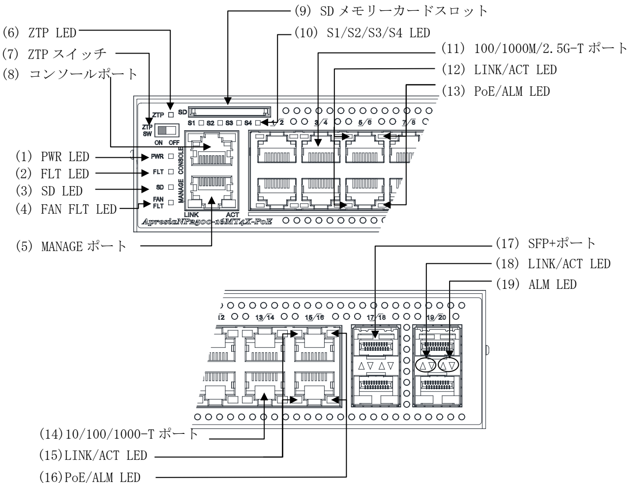
図 2-7 ApresiaNP2500-16MT4X-PoE フロントパネルの構成
