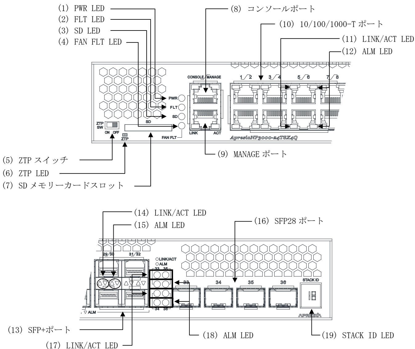
図 2-5 ApresiaNP3000-24T8X4Q フロントパネルの構成
