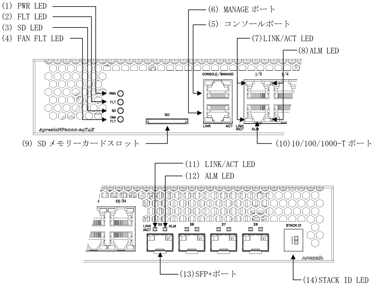
図 2-12 ApresiaNP2000-24T4X フロントパネルの構成
