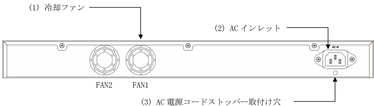
図 2-21 ApresiaNP2100-24T4X、ApresiaNP2100-48T4X、ApresiaNP2000-24T4X、ApresiaNP2000-48T4X のリアパネル
