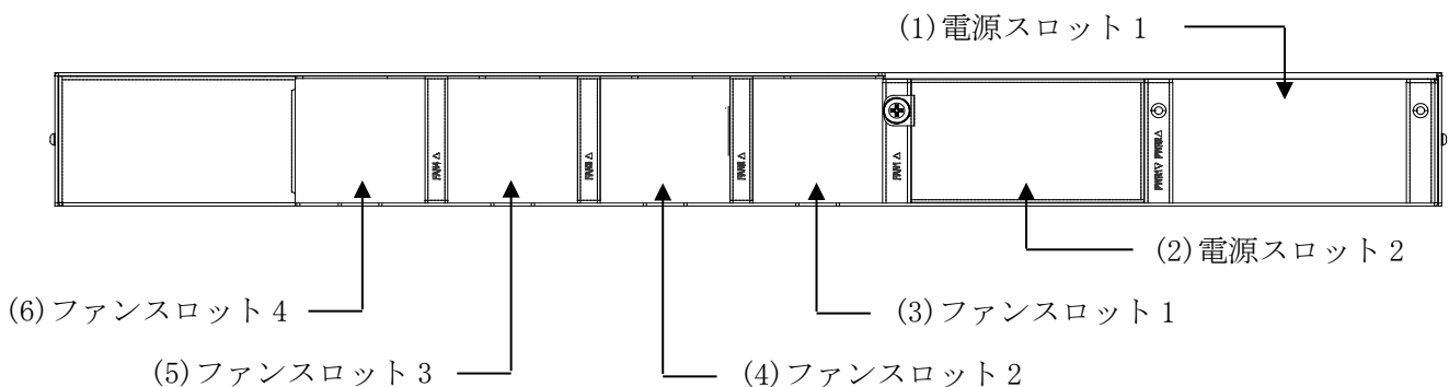
図 2-16 ApresiaNP7000-48X6L、ApresiaNP7000-24G24X6L のリアパネル
