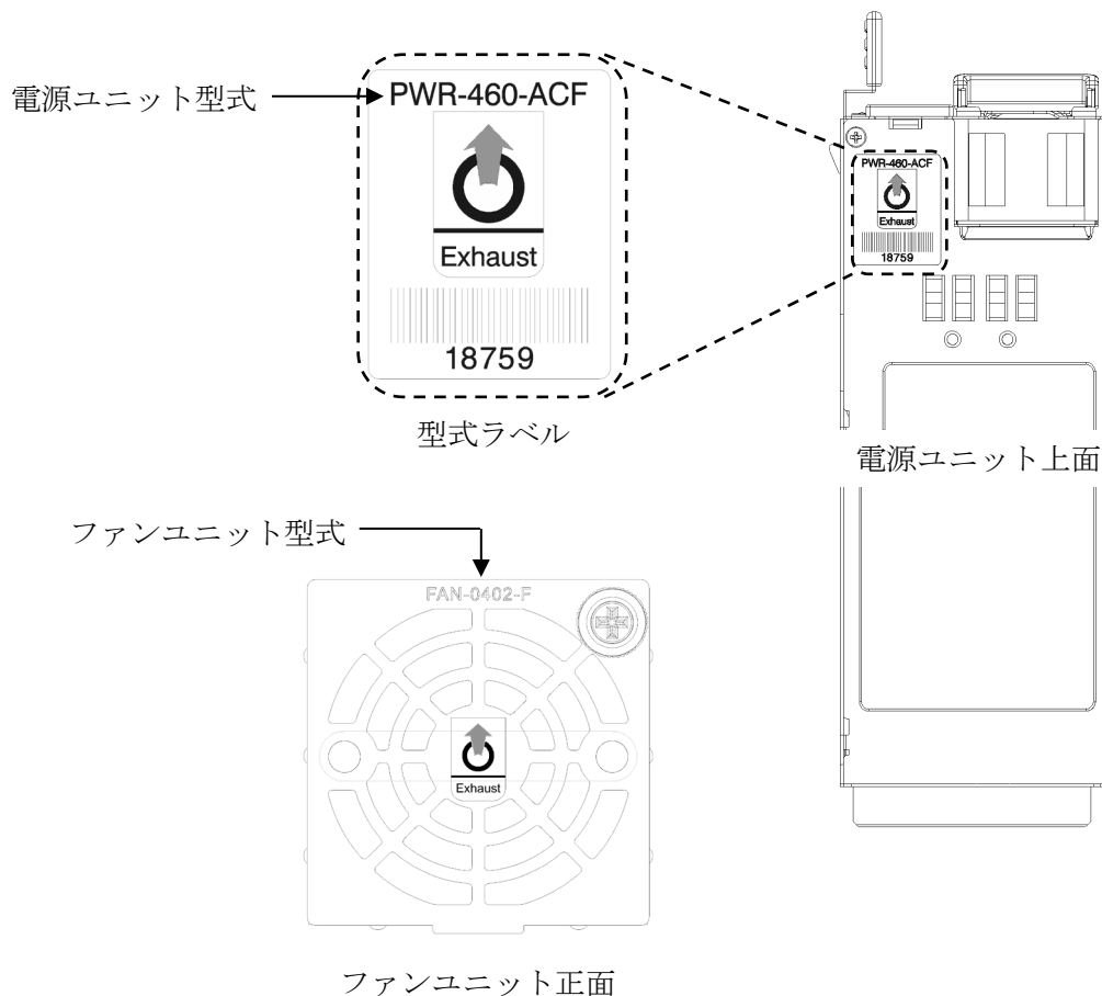
図 3-22 ユニット型式表示
