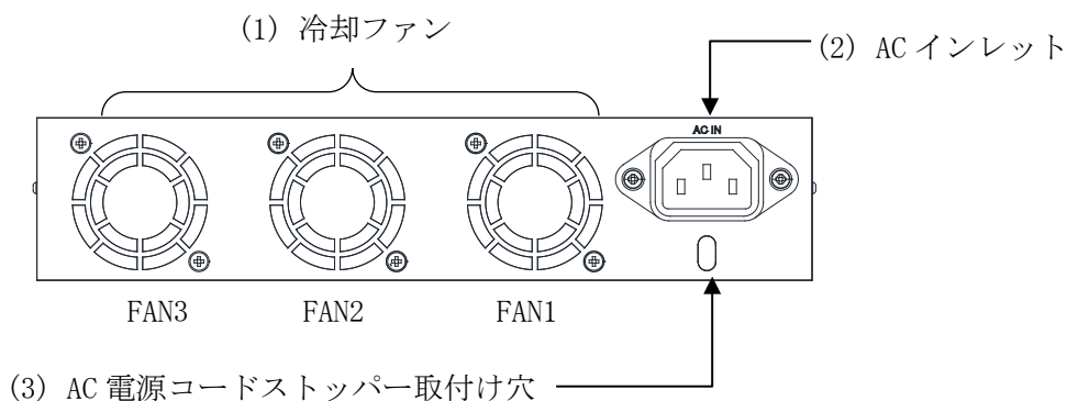
図 2-20 ApresiaNP2500-8MT4X-PoE、ApresiaNP2500-16MT4X-PoE のリアパネル
