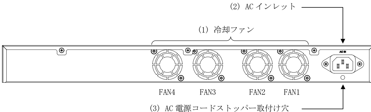
図 2-22 ApresiaNP2100-24T4X-PoE、ApresiaNP2100-48T4X-PoE、ApresiaNP2000-24T4X-PoE、ApresiaNP2000-48T4X-PoE のリアパネル
