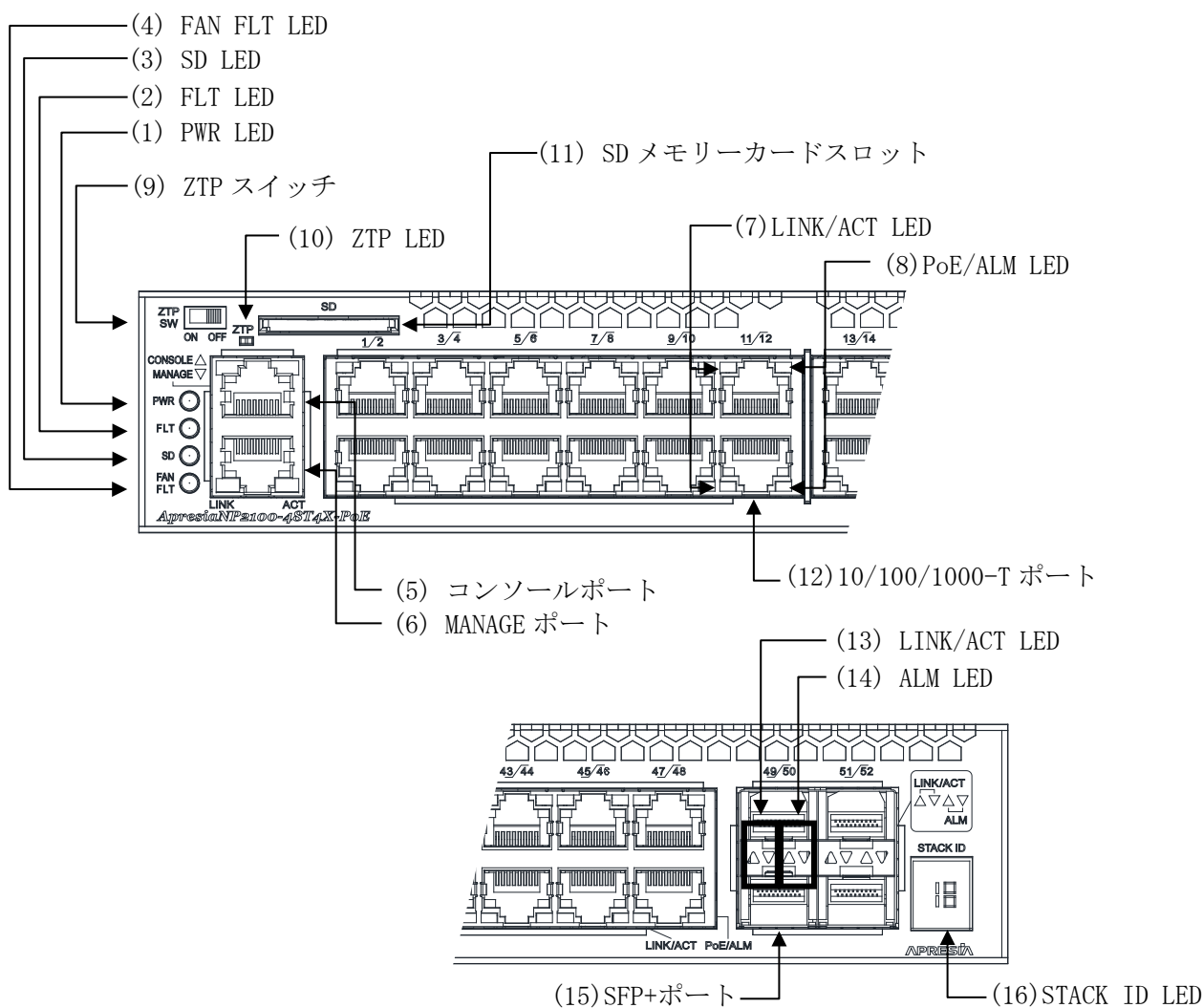
図 2-11 ApresiaNP2100-48T4X-PoE フロントパネルの構成
