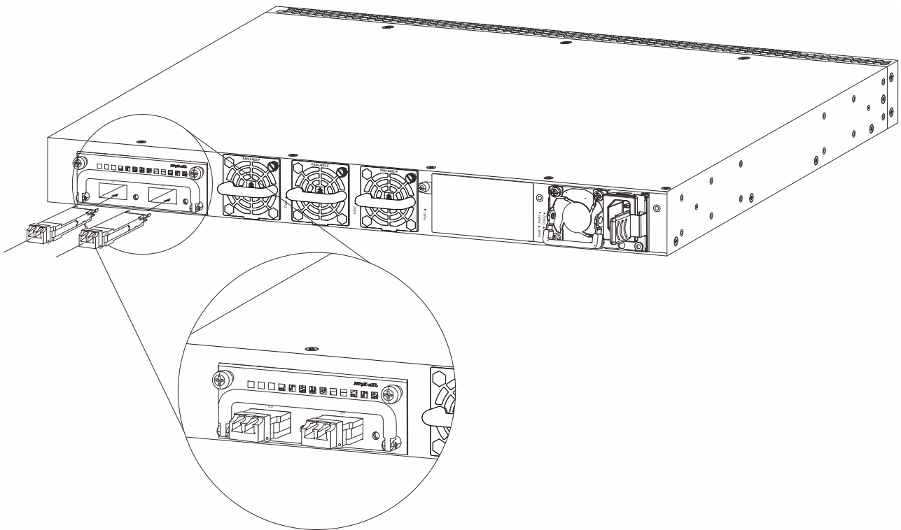
図 3-19 ApresiaNP5000-48T4X QSFP+挿入向き
