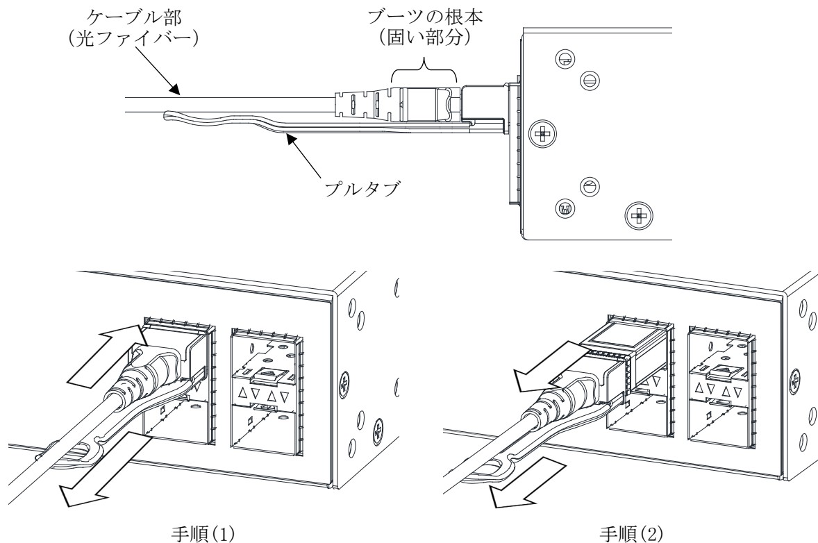
図 3-21 SFP+/SFP28 AOC の取り外し方法 (製品型式 H-SFP+AOCxM の例)
