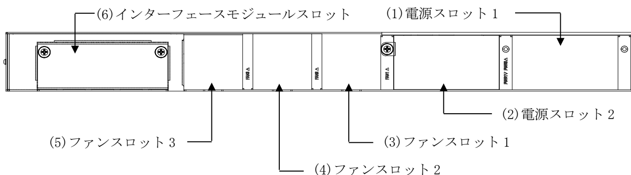
図 2-17 ApresiaNP5000-48T4X のリアパネル
