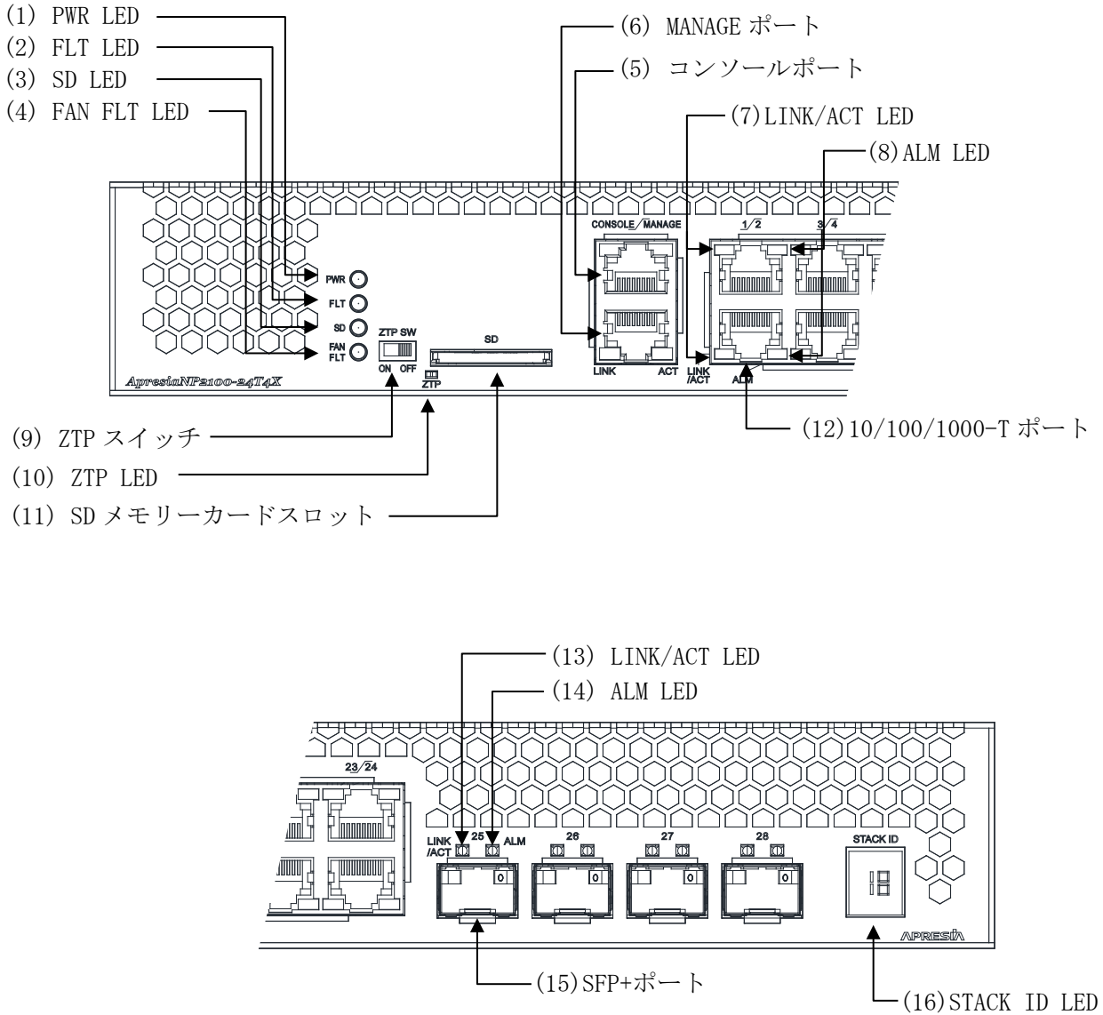
図 2-8 ApresiaNP2100-24T4X フロントパネルの構成
