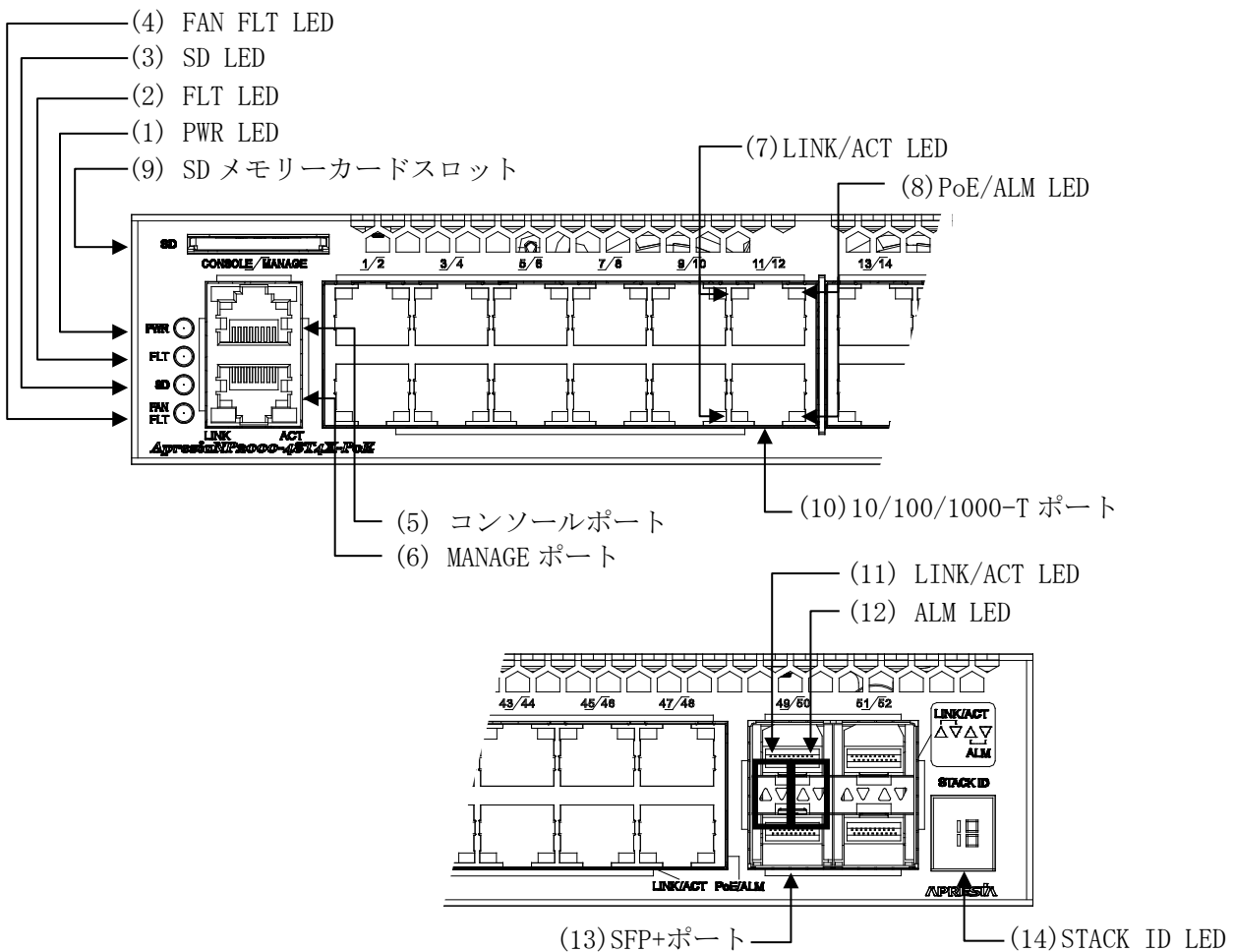
図 2-15 ApresiaNP2000-48T4X-PoE フロントパネルの構成
