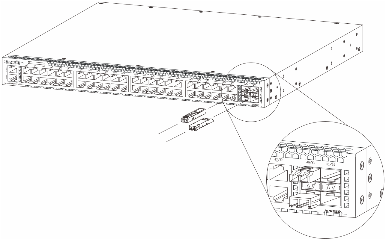
図 3-18 ApresiaNP5000-48T4X、ApresiaNP4000-20Xt4X、ApresiaNP3000-24T8X4Q、ApresiaNP2500-8MT4X-PoE、ApresiaNP2500-16MT4X-PoE、ApresiaNP2100-48T4X、ApresiaNP2100-48T4X-PoE、ApresiaNP2000-48T4X、ApresiaNP2000-48T4X-PoE SFP、SFP+挿入向き
