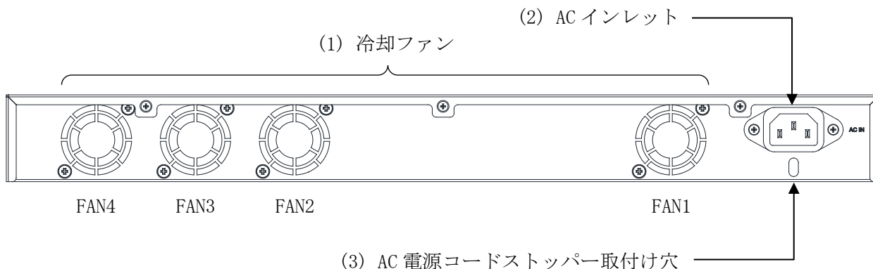
図 2-19 ApresiaN3000-24T8X4Q のリアパネル
