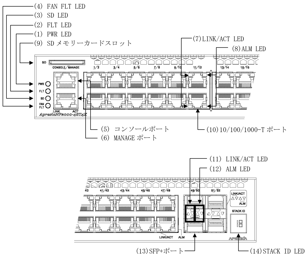
図 2-14 ApresiaNP2000-48T4X フロントパネルの構成
