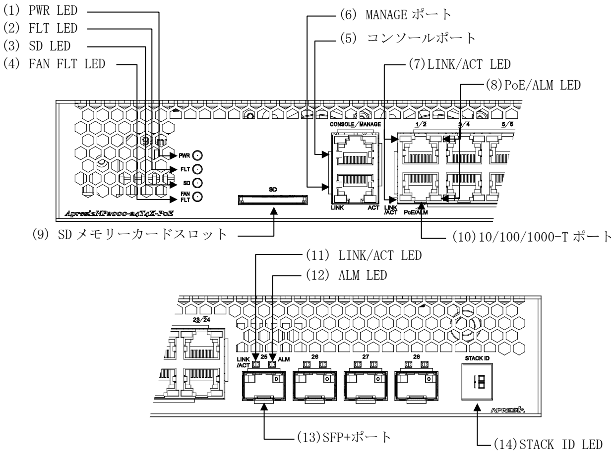
図 2-13 ApresiaNP2000-24T4X-PoE フロントパネルの構成
