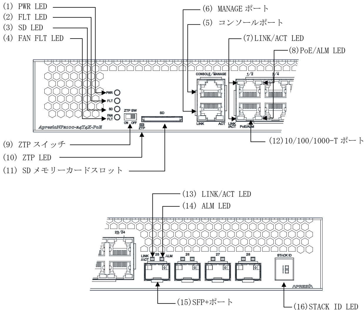
図 2-9 ApresiaNP2100-24T4X-PoE フロントパネルの構成
