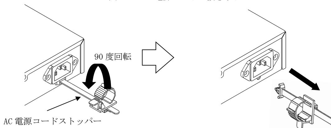
図 3-28 AC 電源コードの抜き取り
