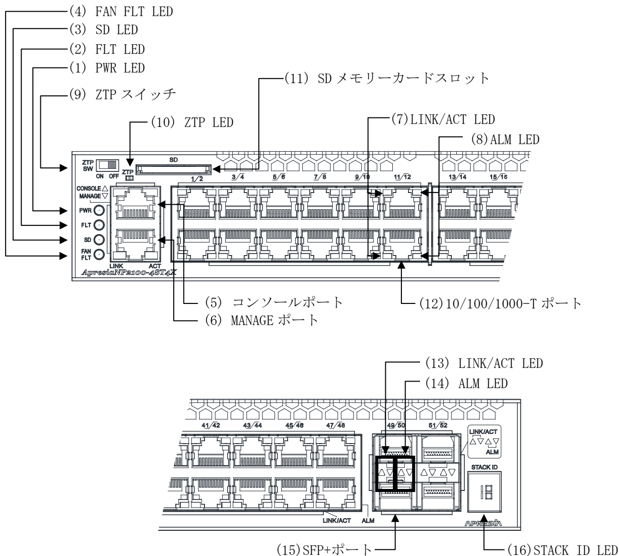
図 2-10 ApresiaNP2100-48T4X フロントパネルの構成
