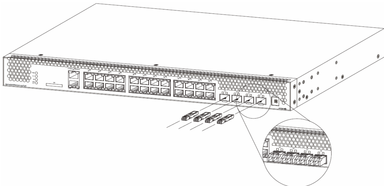
図 3-20 ApresiaNP3000-24T8X4Q、ApresiaNP2100-24T4X、ApresiaNP2100-24T4X-PoE、ApresiaNP2000-24T4X、ApresiaNP2000-24T4X-PoE SFP、SFP+、SFP28 挿入向き
