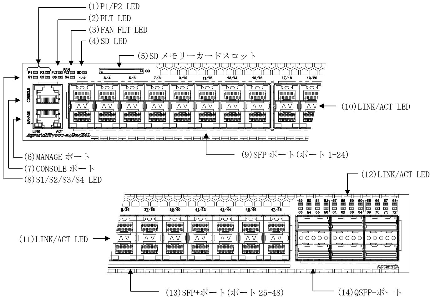
図 2-2 ApresiaNP7000-24G24X6L フロントパネルの構成
