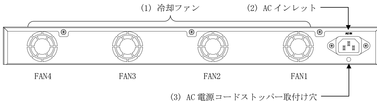
図 2-18 ApresiaNP4000-20Xt4X のリアパネル
