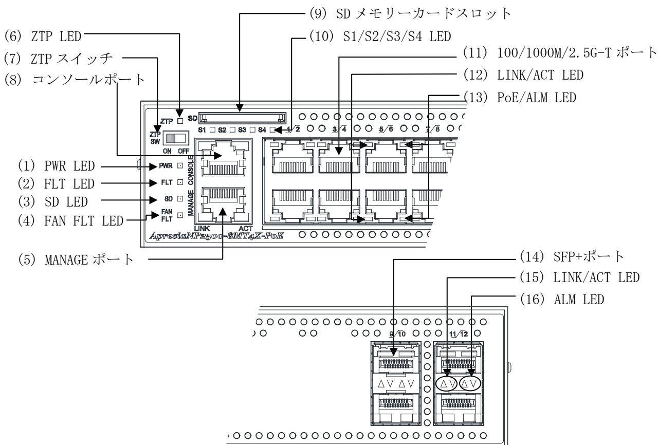
図 2-6 ApresiaNP2500-8MT4X-PoE フロントパネルの構成
