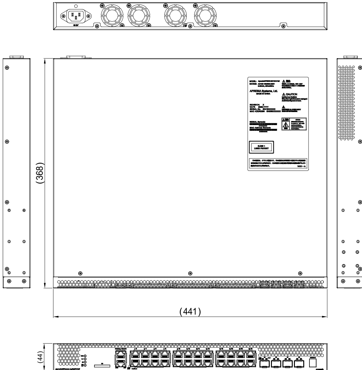
図 10-1 ApresiaNP2000-24T4X-PoE 外観図
