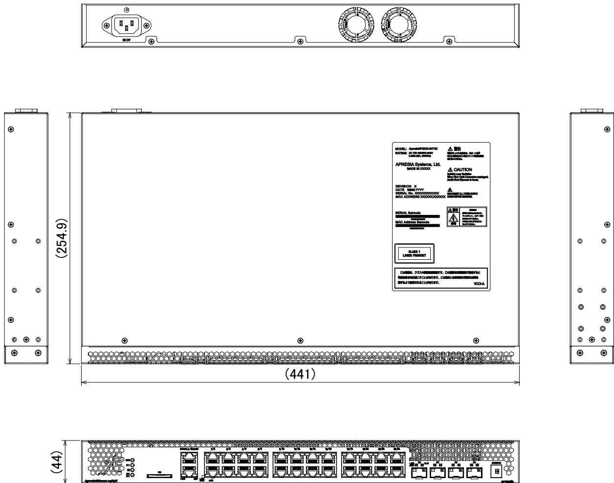
図 10-1 ApresiaNP2000-24T4X 外観図 (Rev. A)
