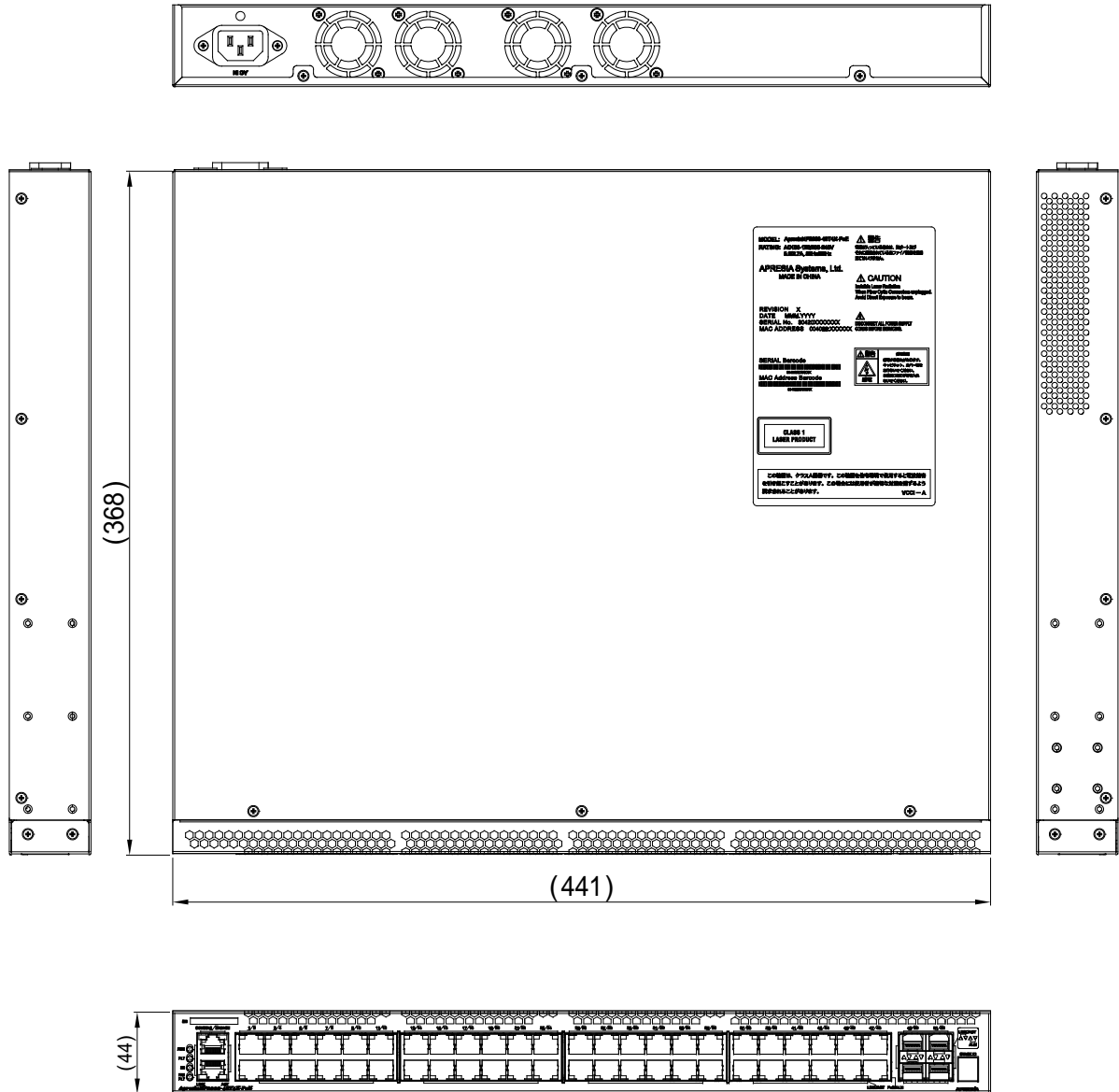
図 10-1 ApresiaNP2000-48T4X-PoE 外観図
