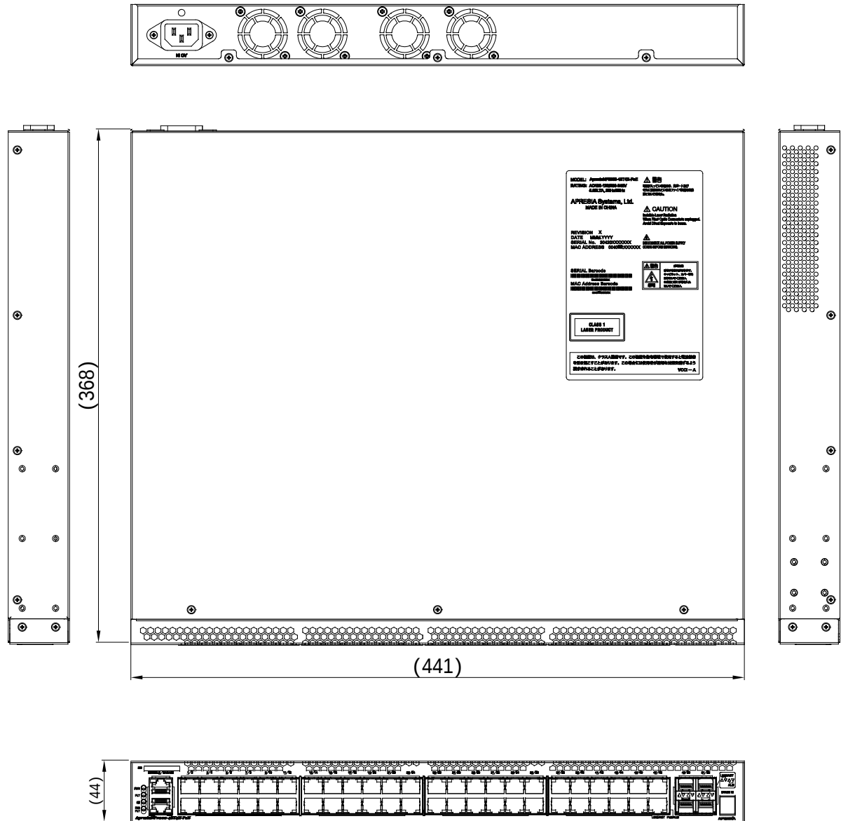
図 10-1 ApresiaNP2000-48T4X-PoE 外観図
