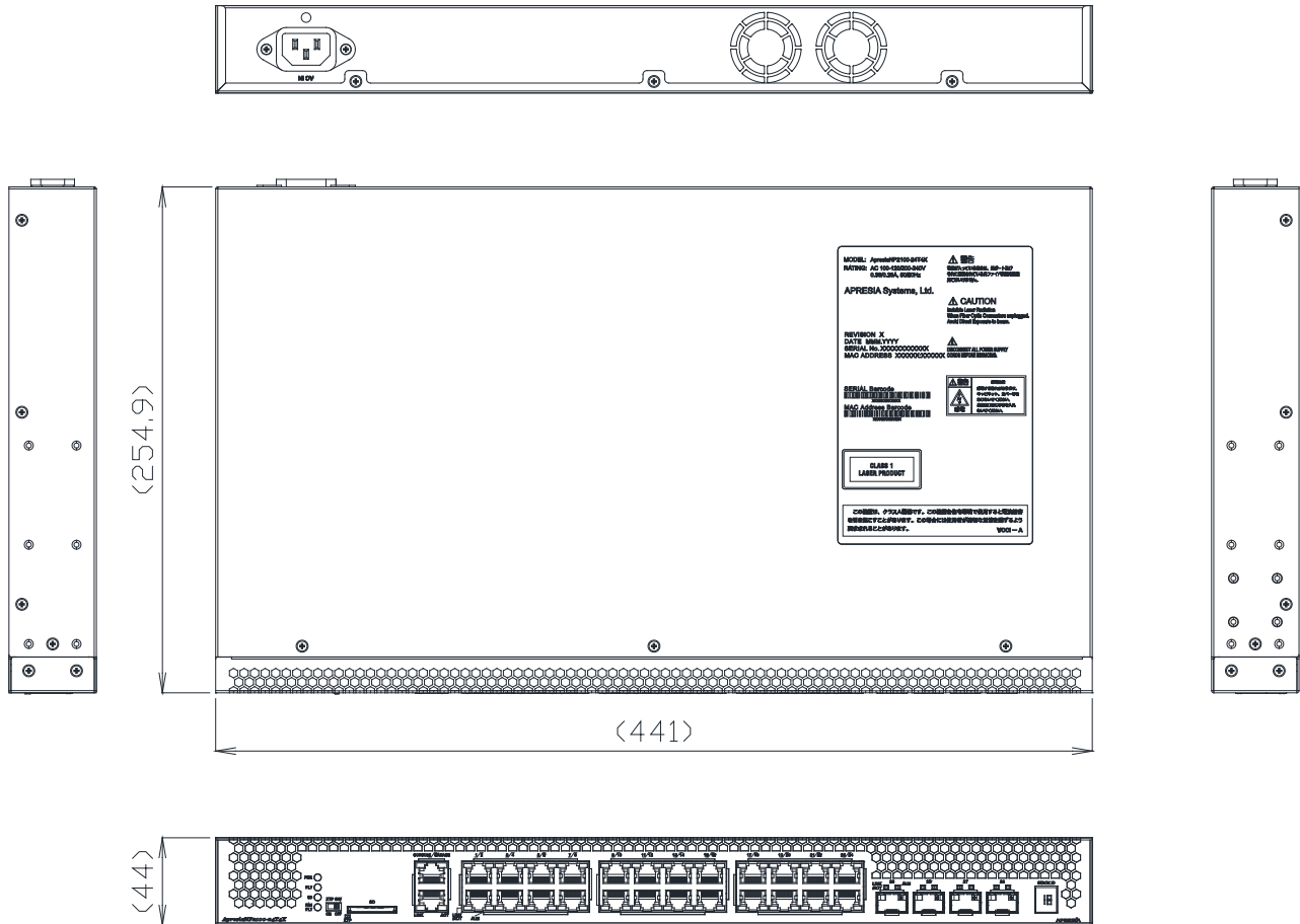
図 10-1 ApresiaNP2100-24T4X 外観図
