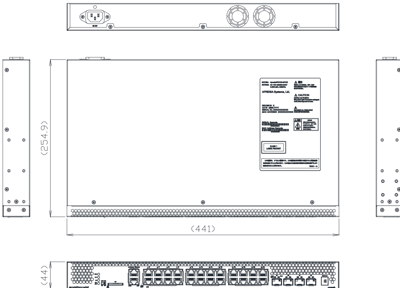
図 10-1 ApresiaNP2100-24T4X 外観図(レビジョン A)
