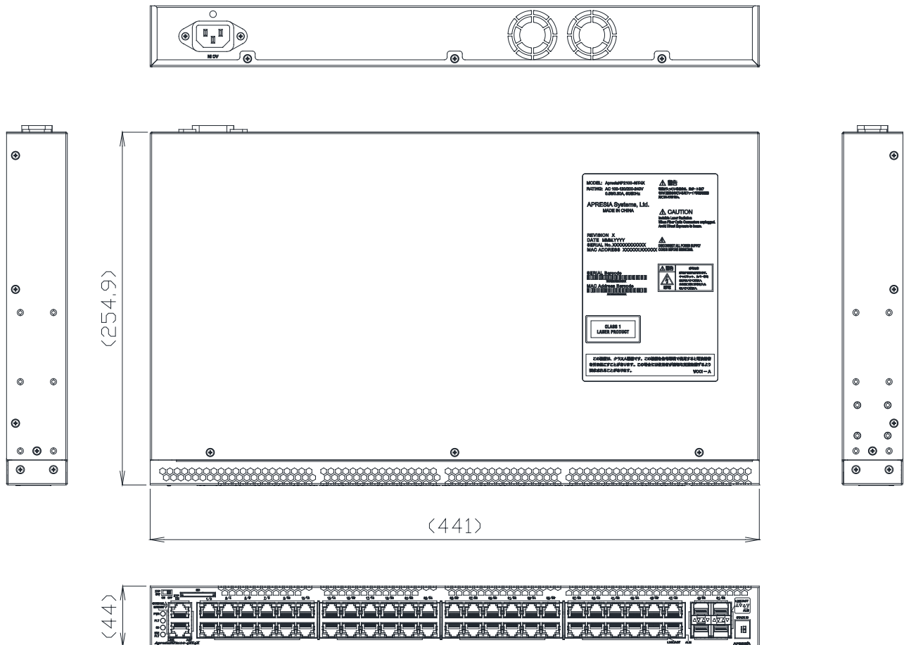
図 10-1 ApresiaNP2100-48T4X 外観図
