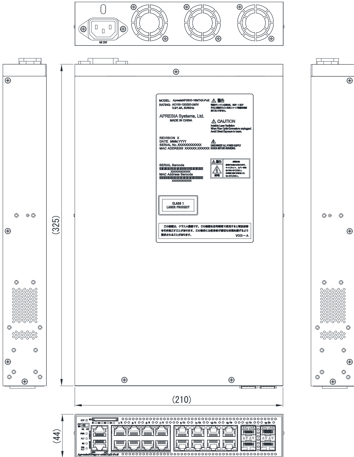
図 10-1 ApresiaNP2500-16MT4X-PoE 外観図
