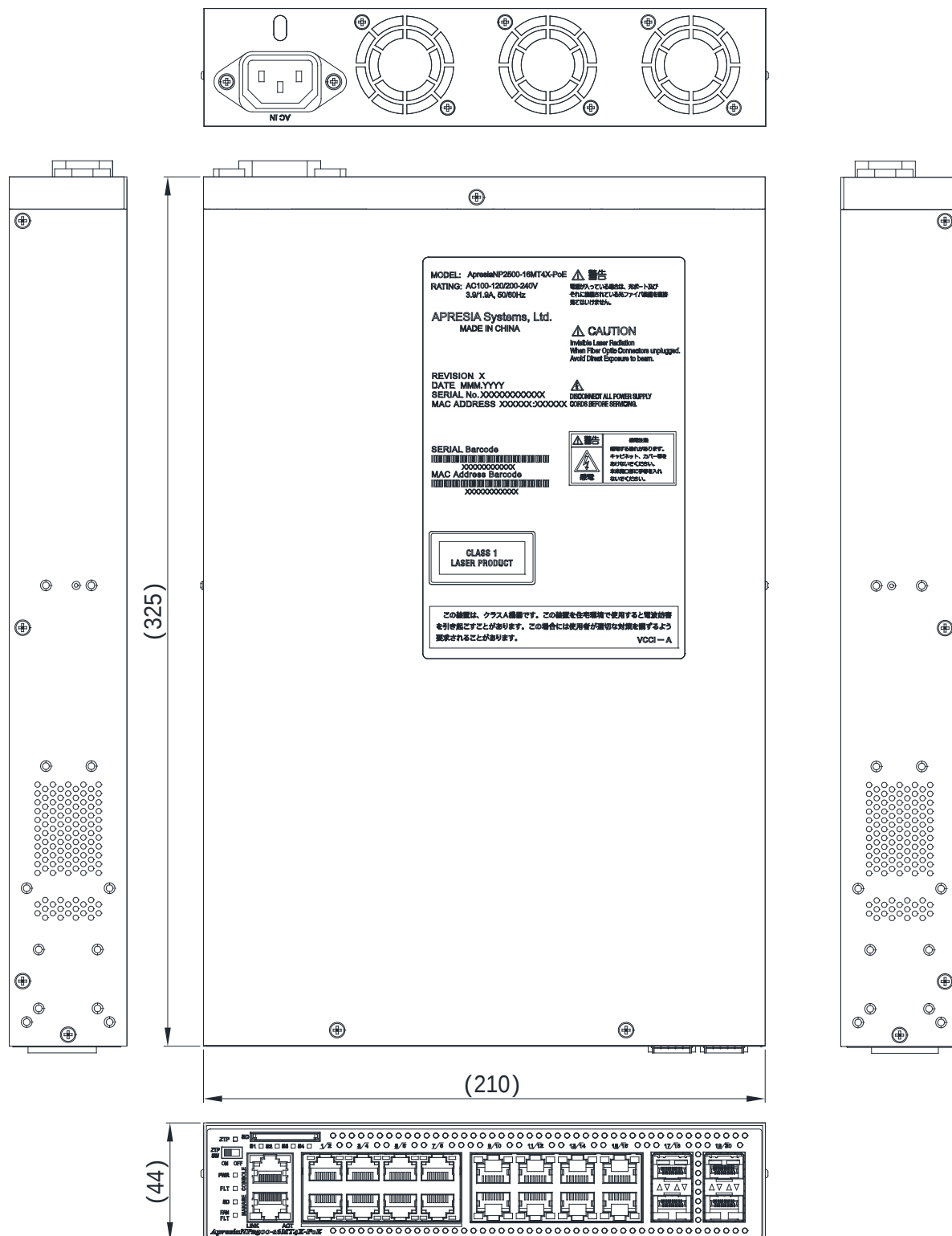
図 10-1 ApresiaNP2500-16MT4X-PoE 外観図
