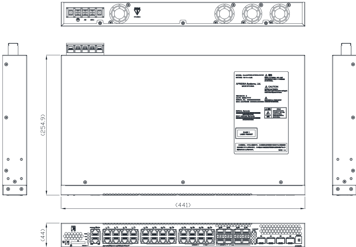
図 10-1 ApresiaNP3000-24T8X4Q-DC110V 外観図
