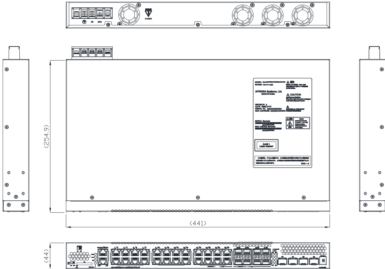
図 10-1 ApresiaNP3000-24T8X4Q-DC110V 外観図
