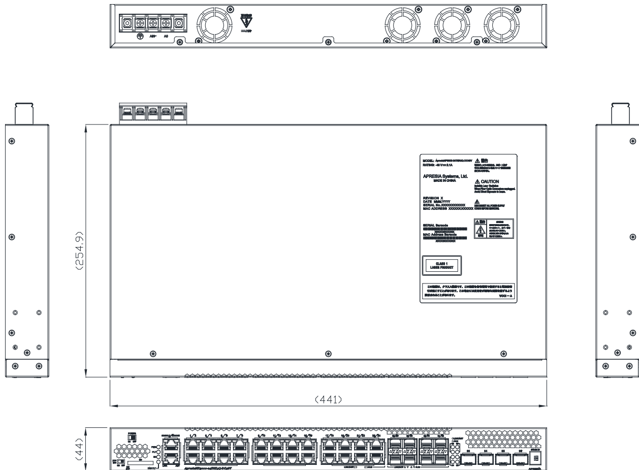
図 10-1 ApresiaNP3000-24T8X4Q-DC48V 外観図
