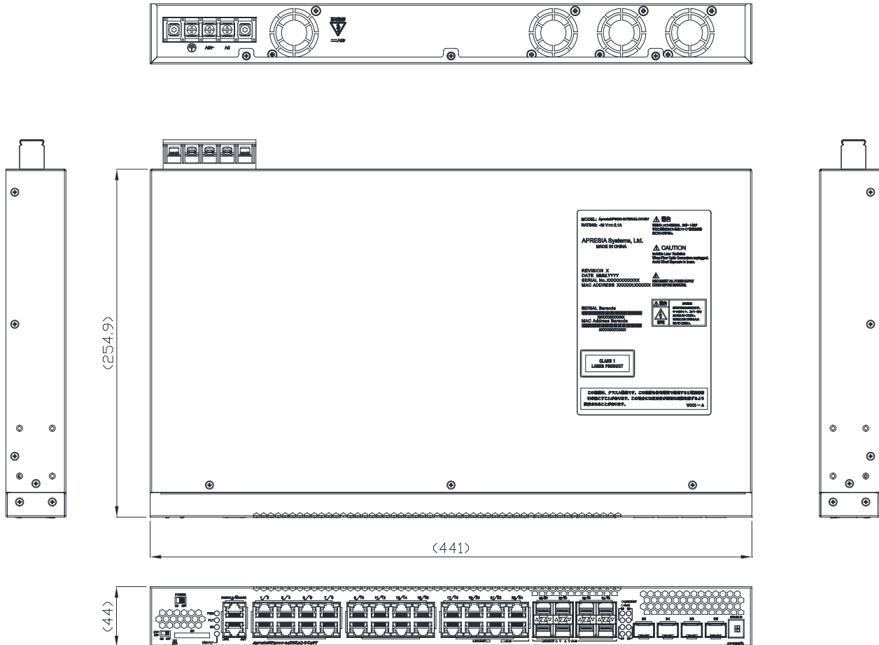
図 10-1 ApresiaNP3000-24T8X4Q-DC48V 外観図
