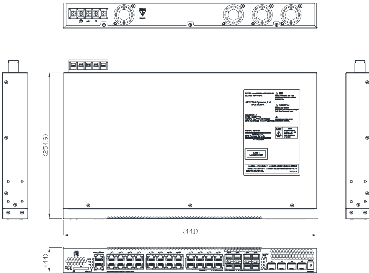
図 10-1 ApresiaNP3000-24T8X4Q-DC48V 外觀図
