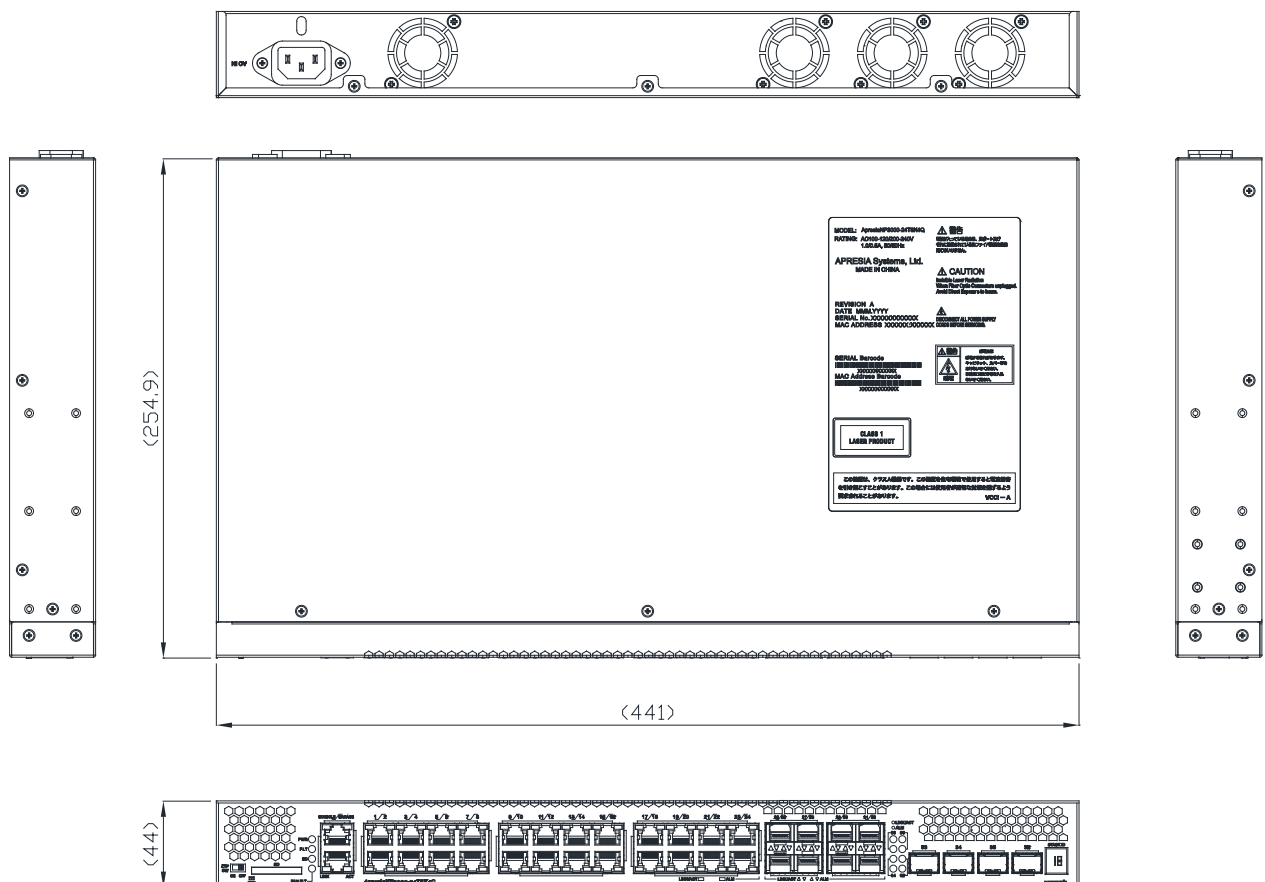
図 10-1 ApresiaNP3000-24T8X4Q 外観図
