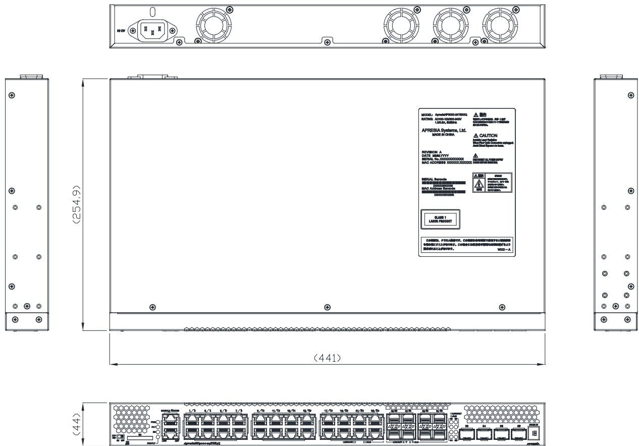
図 10-1 ApresiaNP3000-24T8X4Q 外観図
