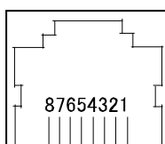
図 6-1 コンソールポートのピン No.
