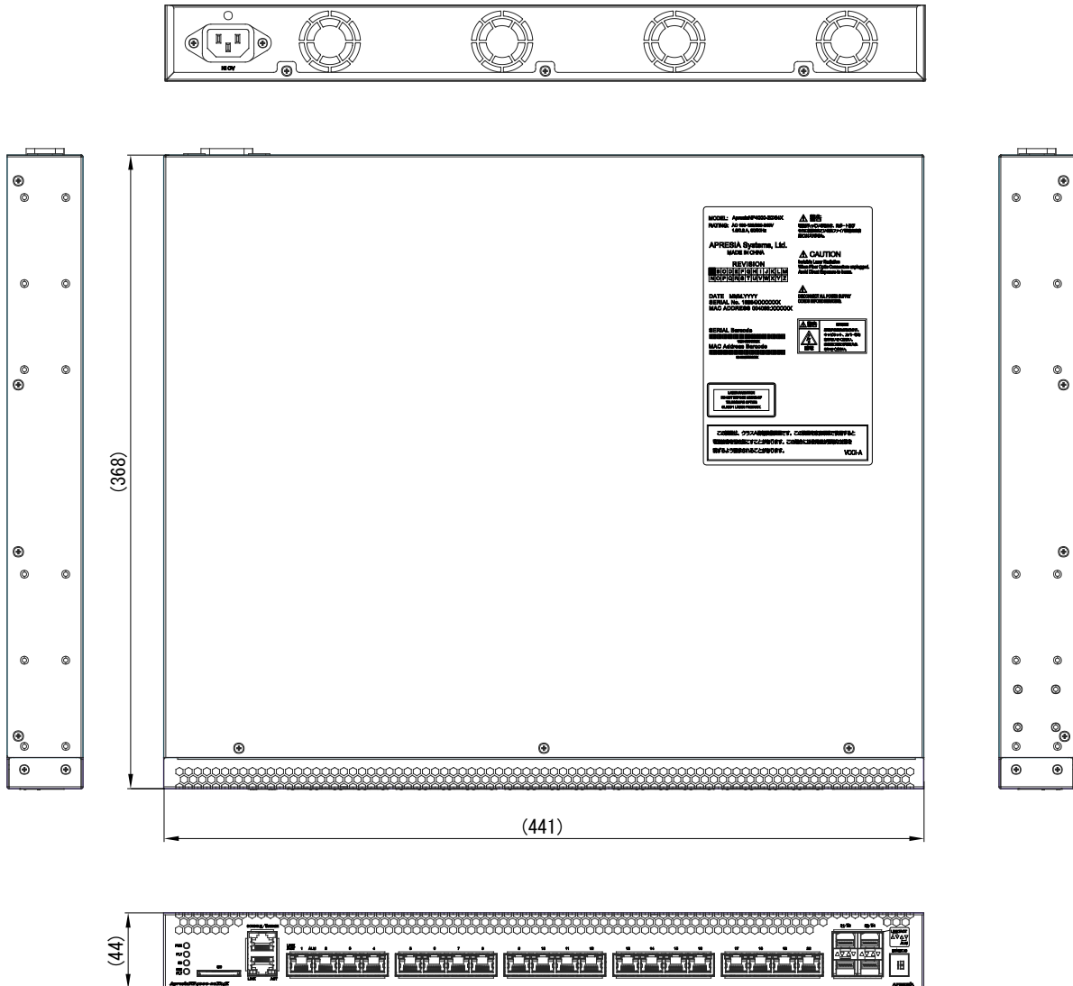
図 10-1 ApresiaNP4000-20Xt4X 外観図 (Rev. A)
