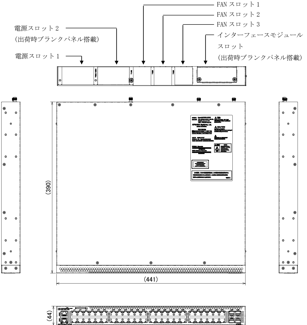
図 10-1 ApresiaNP5000-48T4X 外観図 (Rev. A)
