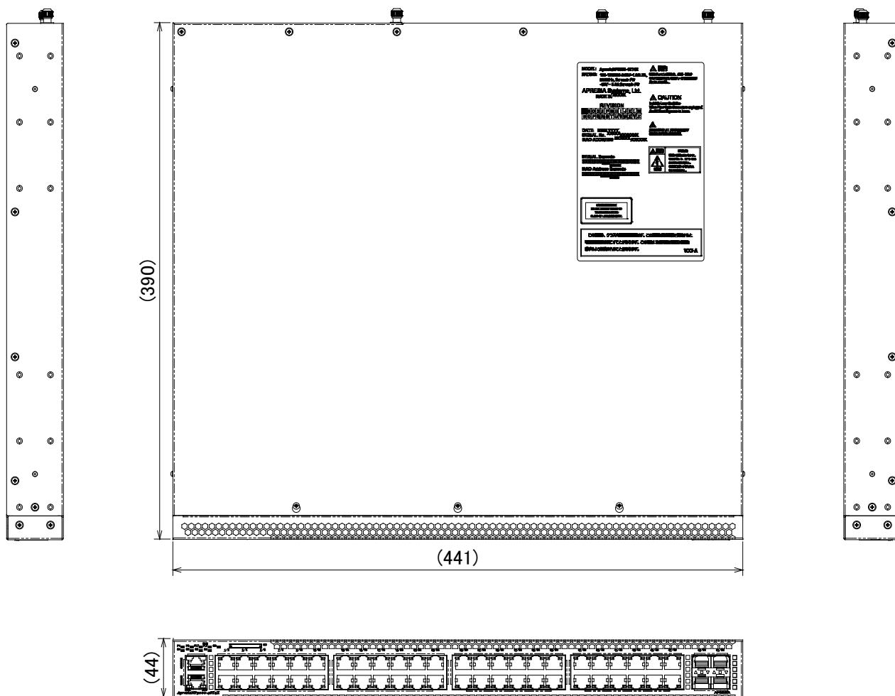
図 10-1 ApresiaNP5000-48T4X 外観図 (Rev. A)
