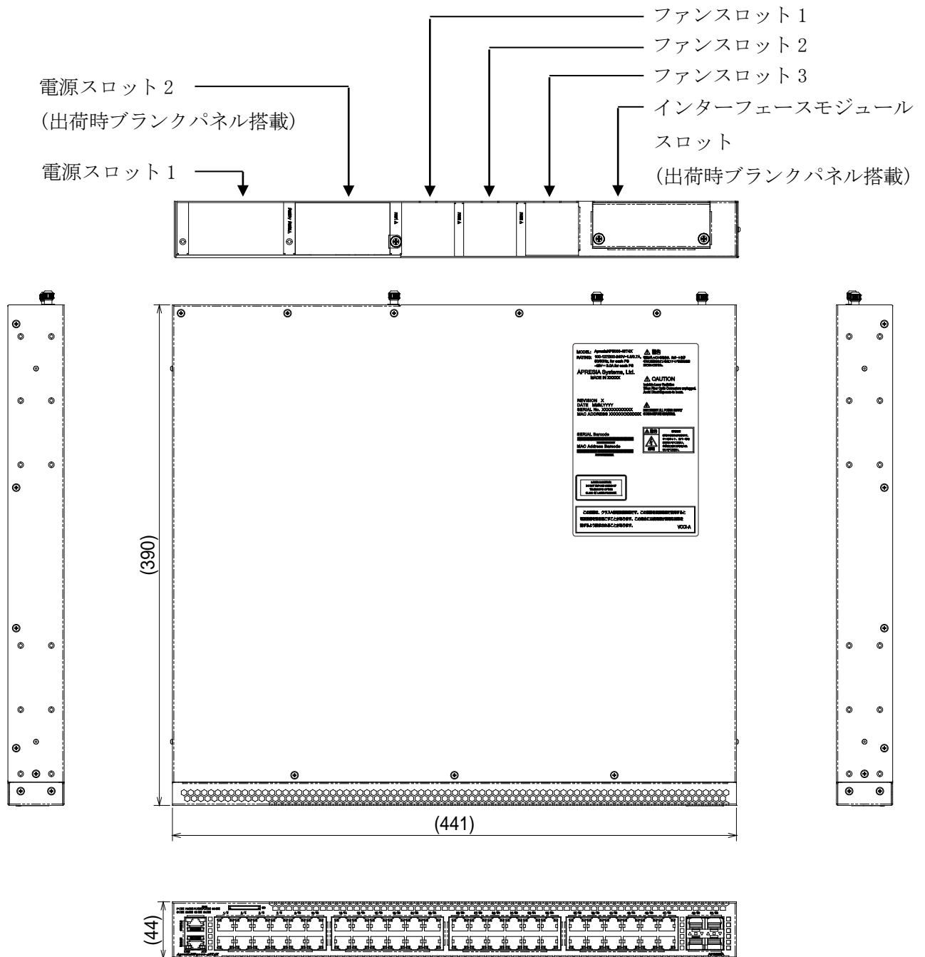
図 10-1 ApresiaNP5000-48T4X 外観図
