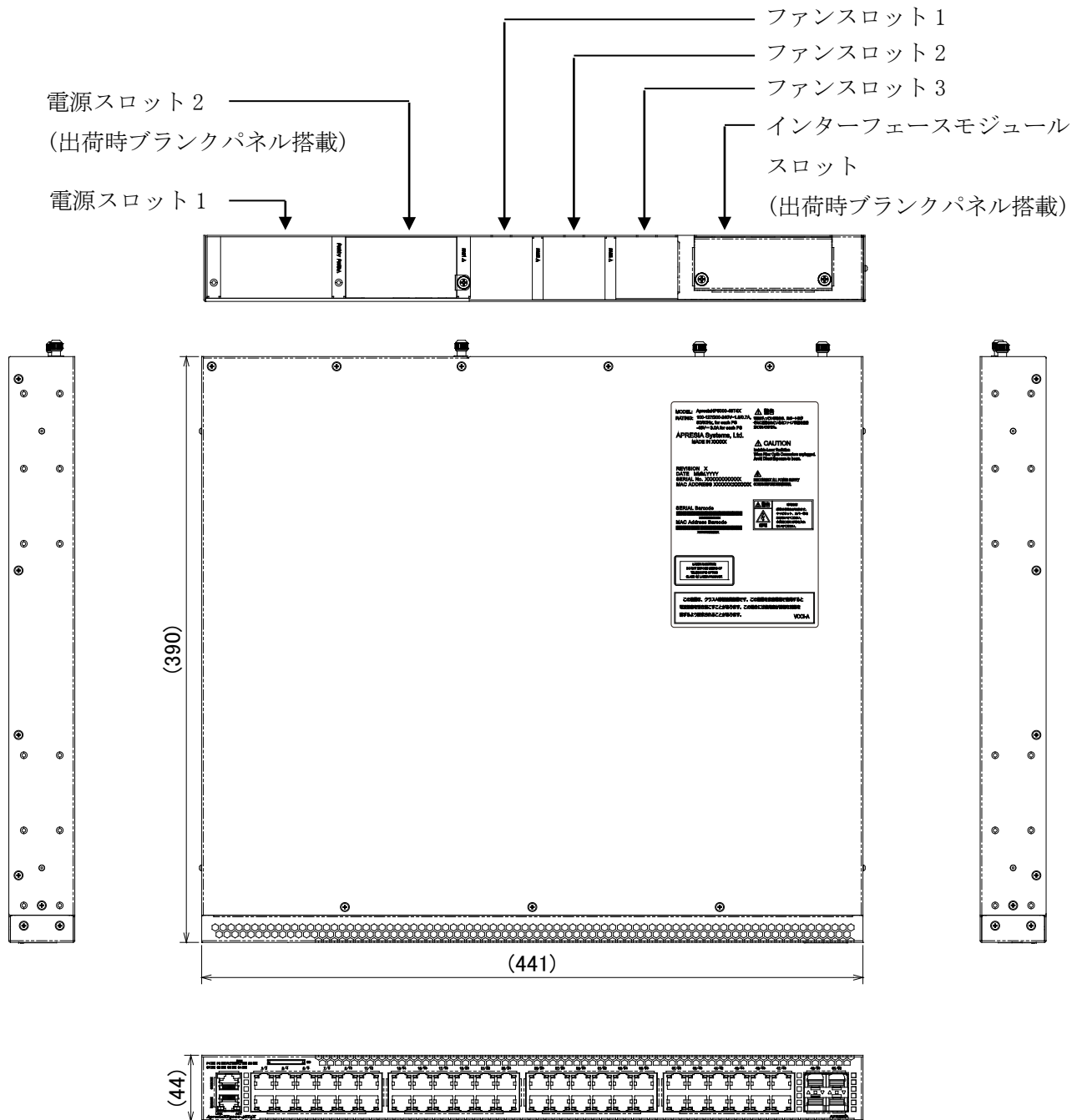
図 10-1 ApresiaNP5000-48T4X 外観図
