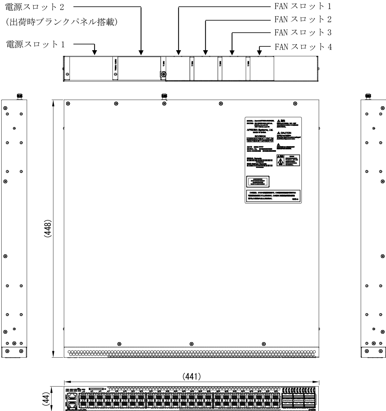
図 10-1 ApresiaNP7000-24G24X6L 外観図 (Rev. A)
