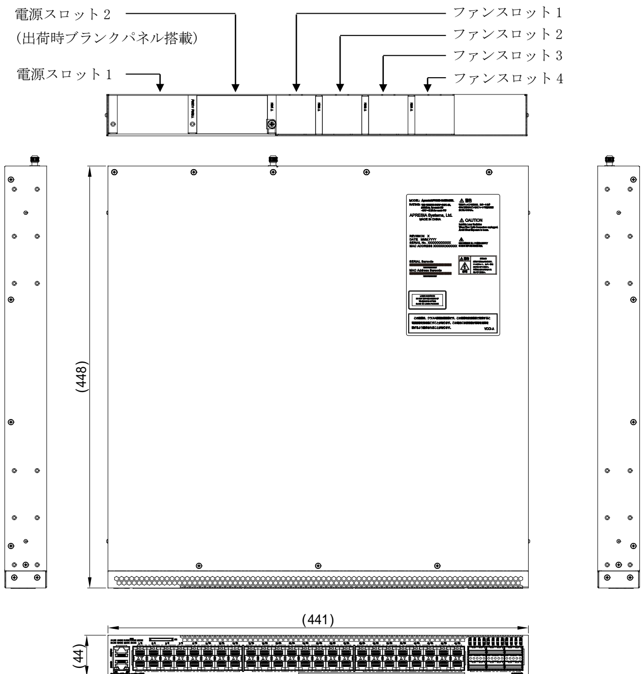
図 10-1 ApresiaNP7000-24G24X6L 外観図
