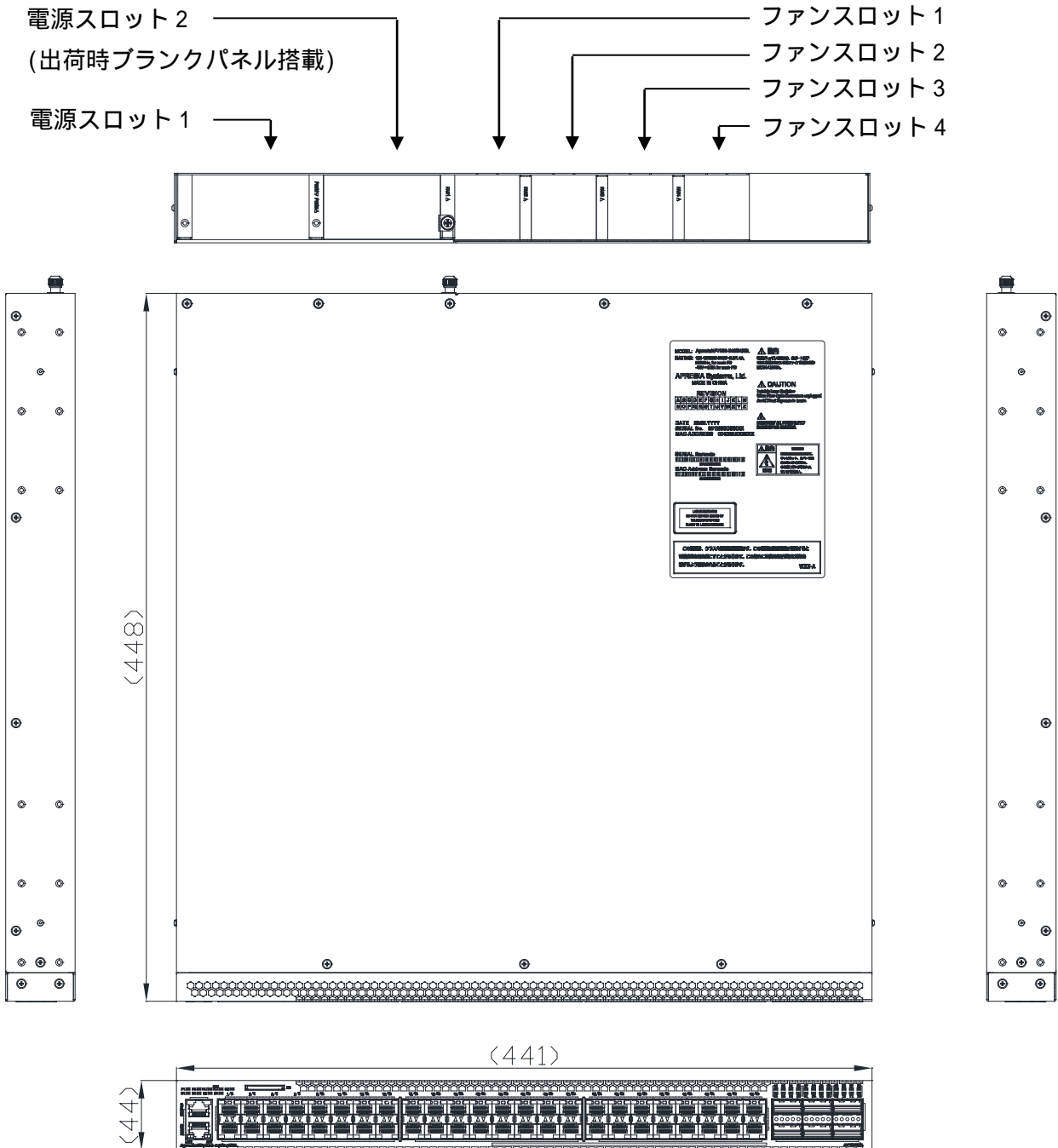
図 10-1 ApresiaNP7000-24G24X6L 外観図
