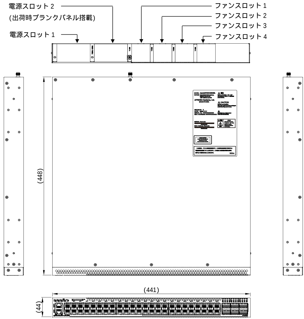
図 10-1 ApresiaNP7000-24G24X6L 外観図
