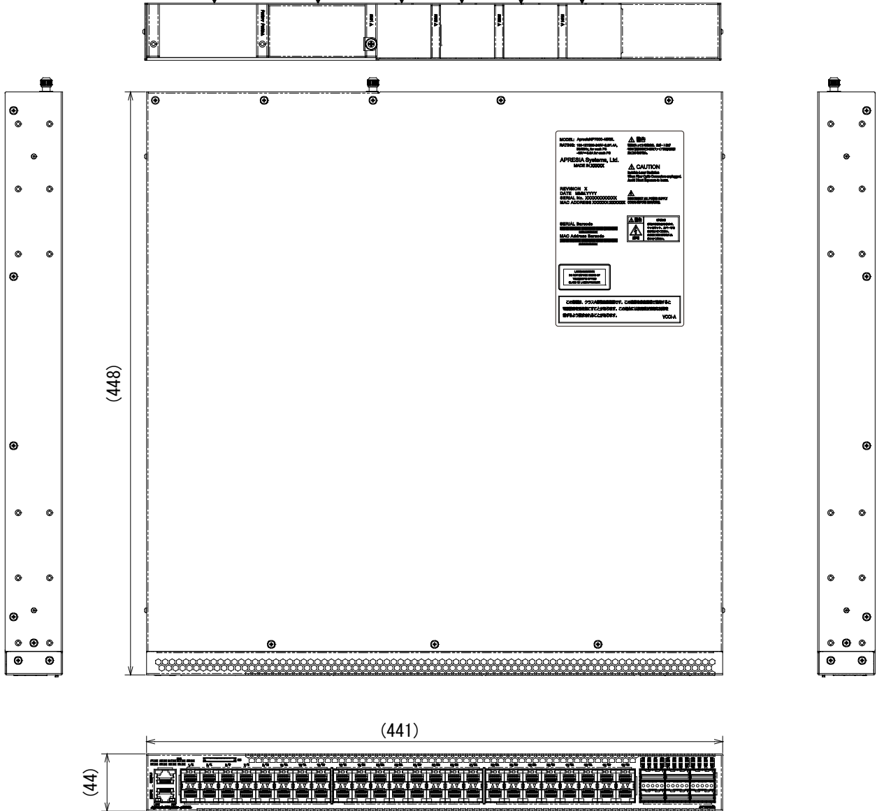
図 10-1 ApresiaNP7000-48X6L 外観図 (Rev. A)
