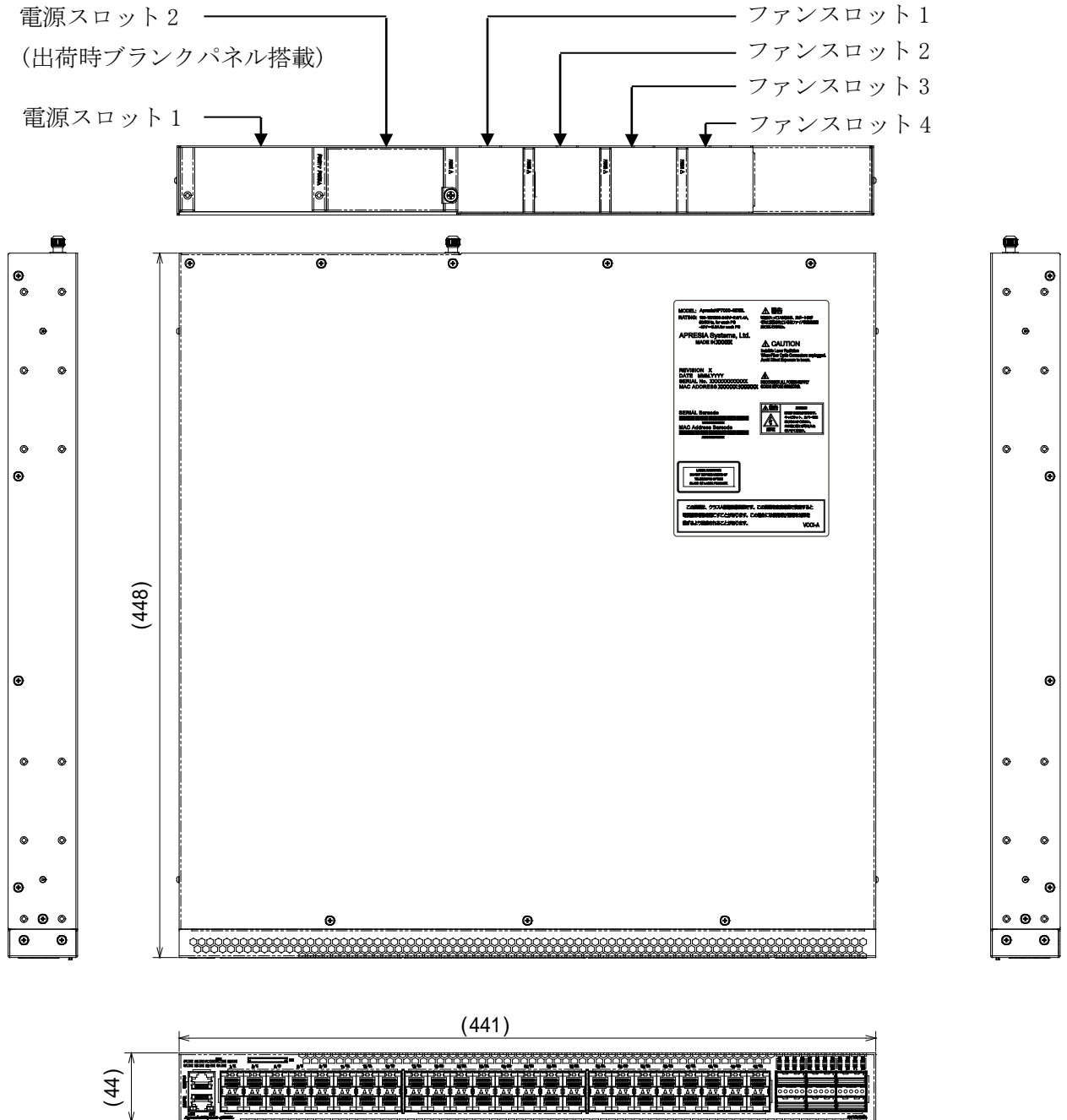
図 10-1 ApresiaNP7000-48X6L 外観図
