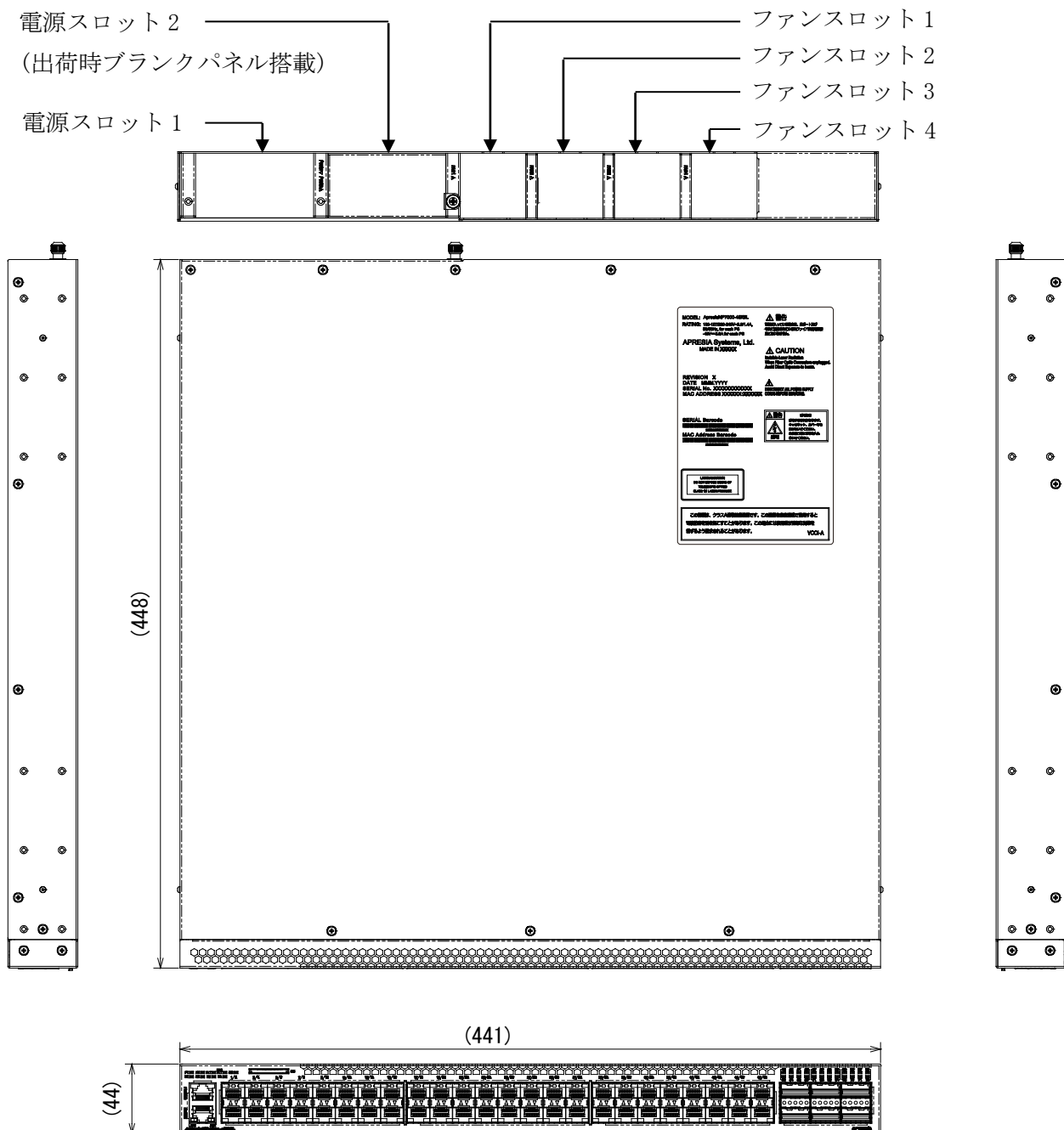
図 10-1 ApresiaNP7000-48X6L 外観図
