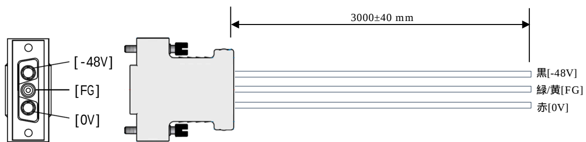
図 8-2 AN-DCPC-3M-01 外観図
