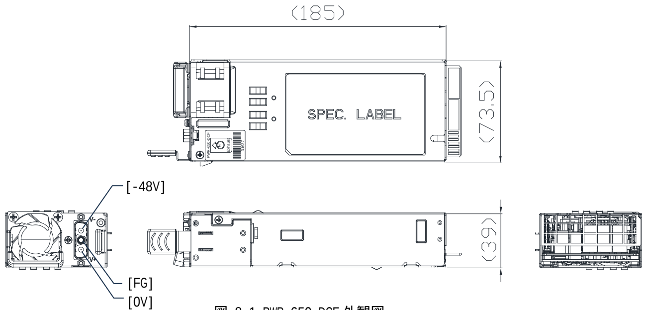
図 8-1 PWR-650-DCF 外観図
