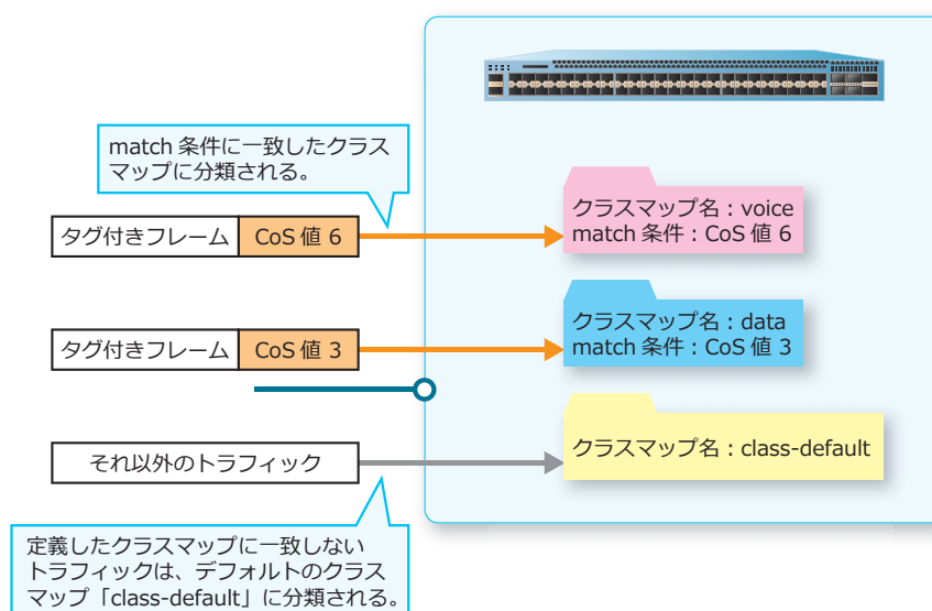
図 11-5 ポリシーマップでの「トラフィックの分類」の例
