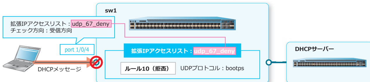
図 8-21 DHCP サーバー宛ての DHCP パケットを破棄する場合の構成例
