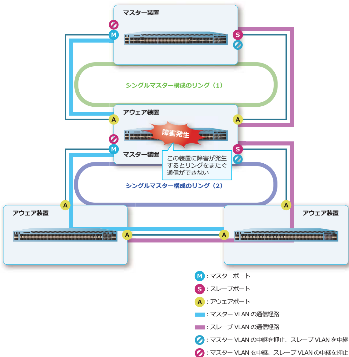
図 14-7 シングルマスター構成の多段接続の例
