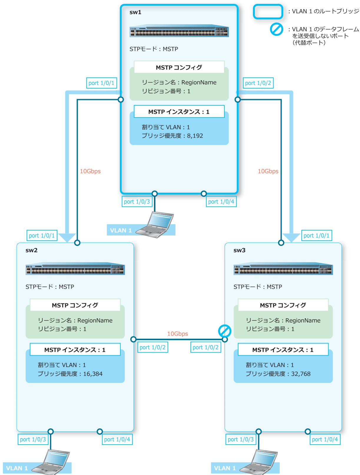
図 5-19 MSTP を使用した場合の設定結果例（MSTP インスタンス 1）
