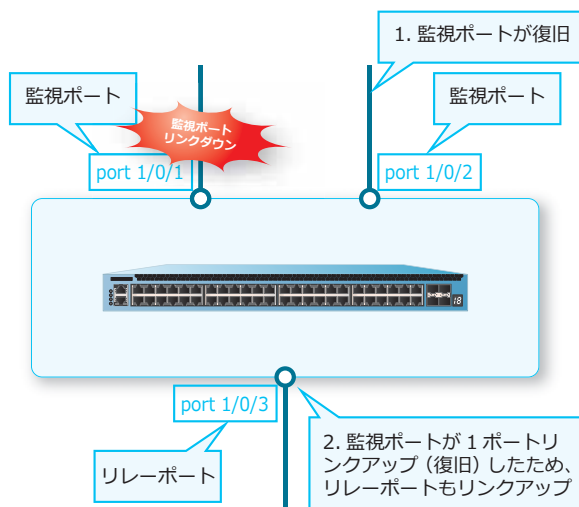
図 15-2 監視ポート復旧時の動作
