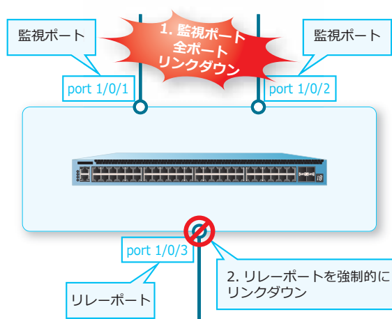
図 15-1 監視ポート障害時の動作
