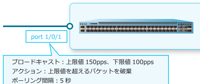
図 7-2 ストームコントロールの設定例
