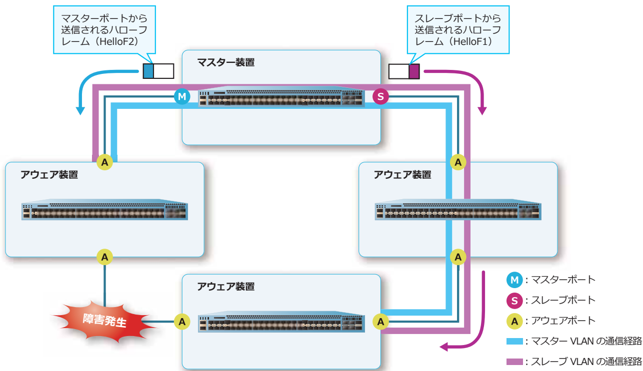
図 14-12 切り替わり後のリングの動作例
