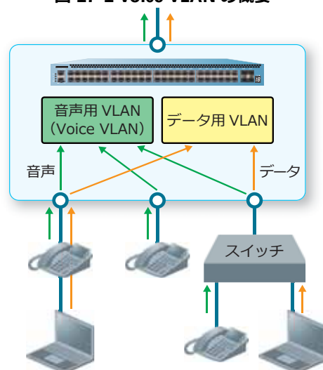
図 17-1 Voice VLAN の概要
