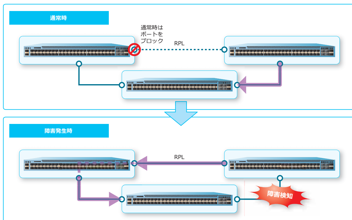
図 10-1 ERPS の概要
