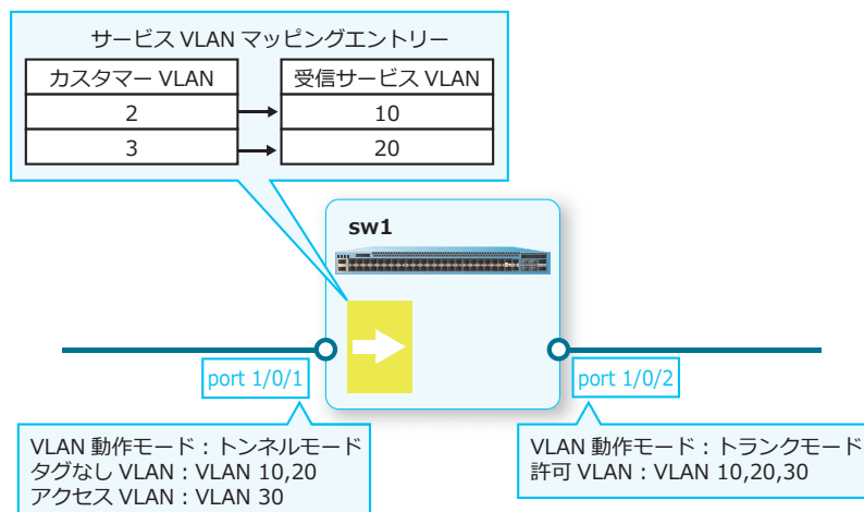
図 4-13 サービス VLAN マッピングエントリーを使用する場合の構成例
