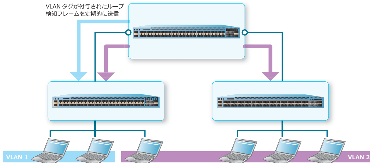
図 6-6 VLAN ベースモードでのループ検知フレームの送信
