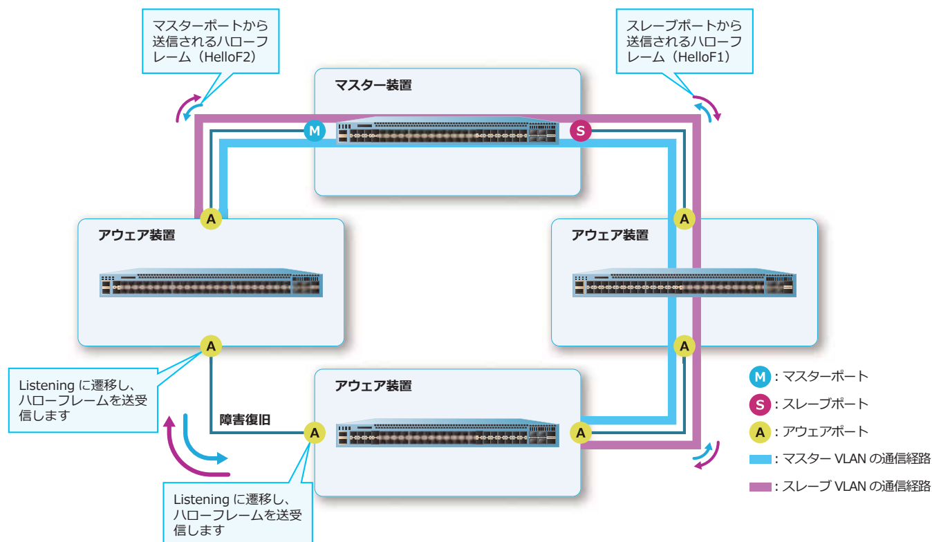
図 14-16 障害復旧時の動作例（1）
