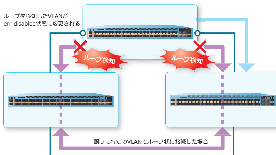
図 6-3 VLAN ベースモードでループを検知した場合
