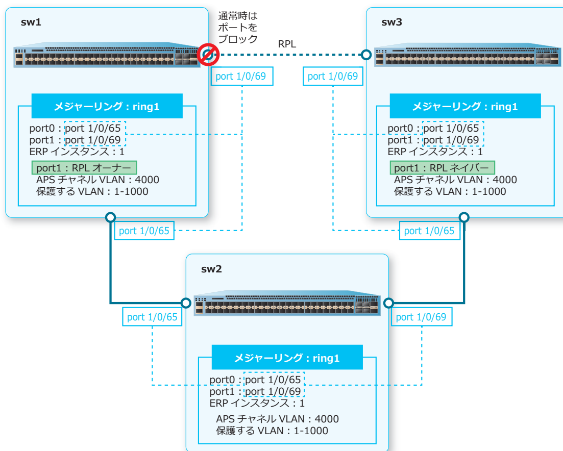
図 10-6 RPL ネイバーの設定例 (sw3)
