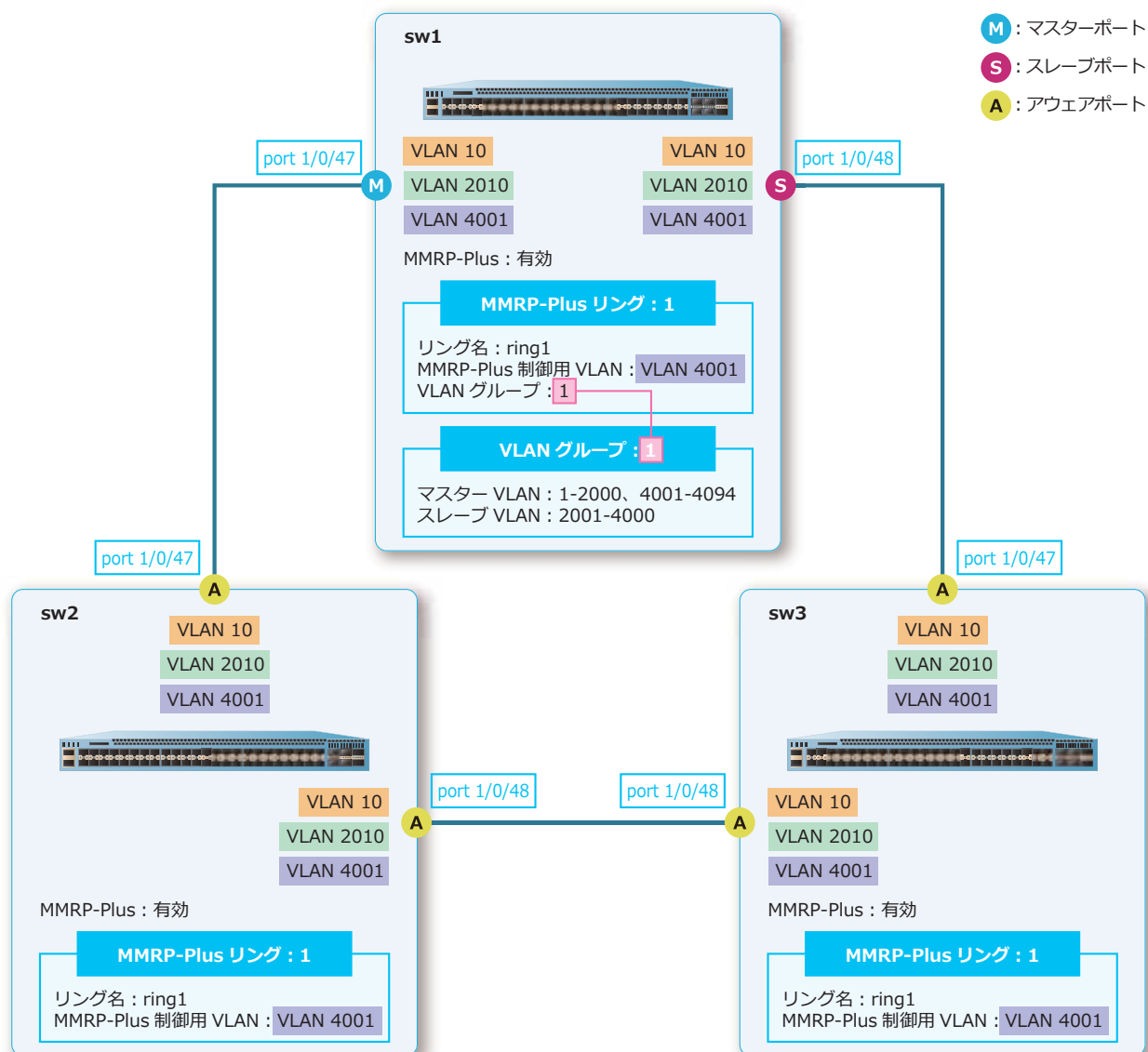
図 14-36 アウエア装置の設定例 (sw2、sw3)
