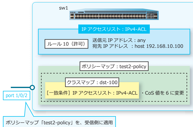
図 11-20 ポリシーマップによるリマーケティングの構成例
