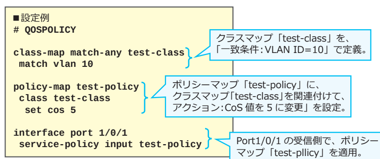
図 11-6 ポリシーマップの設定コマンドの例
