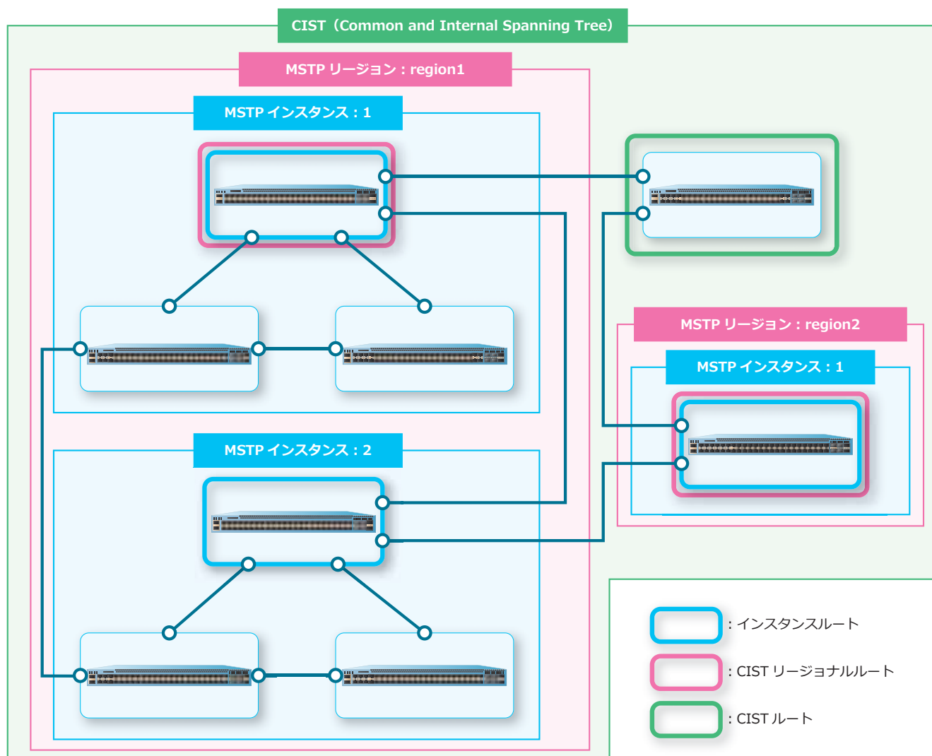
図 5-7 MSTP の概要
