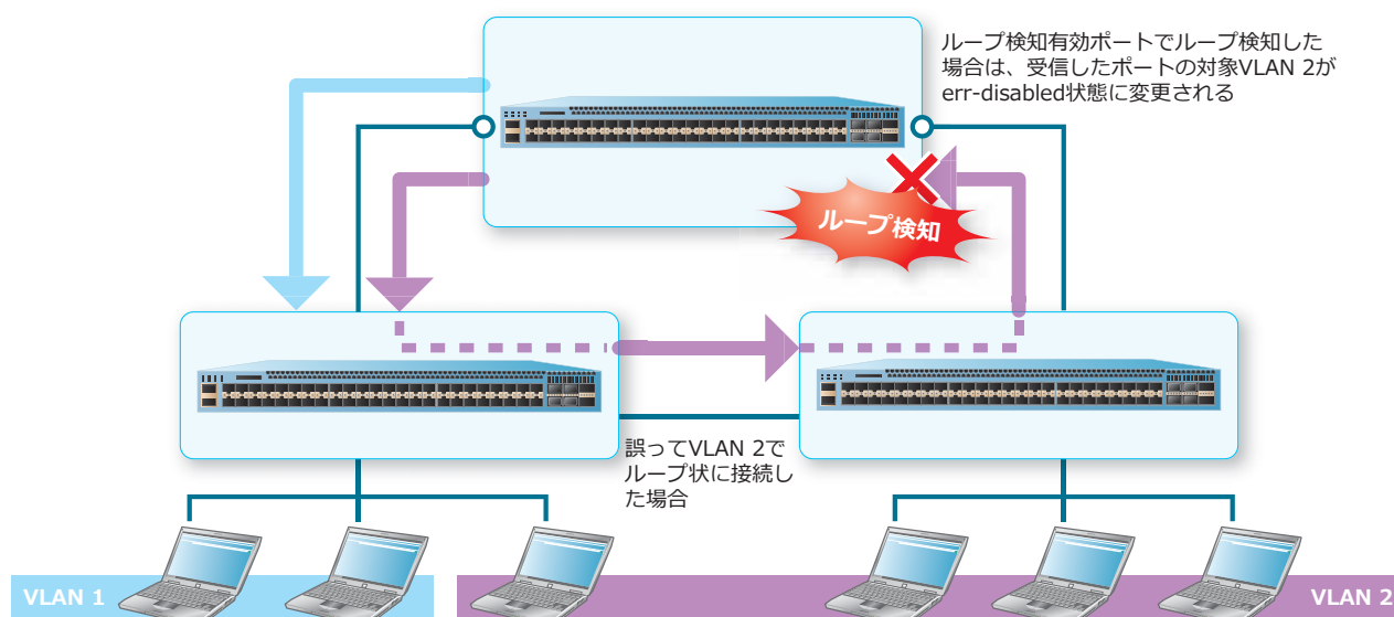
図 6-7 VLAN ベースモードでループを検知した場合
