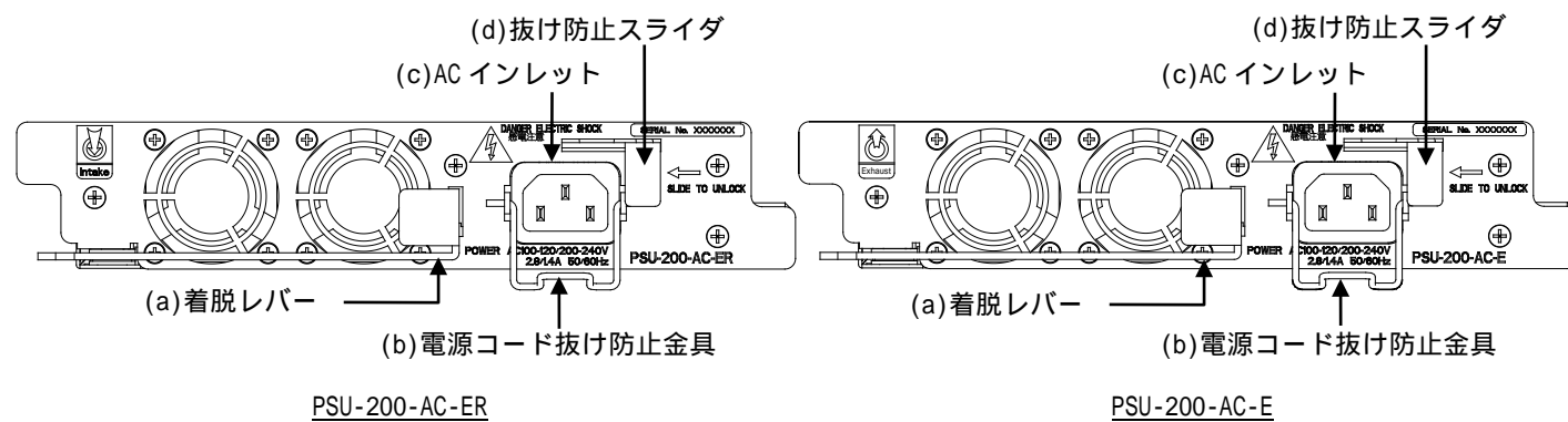
図 1 ユニットの各部の名称
