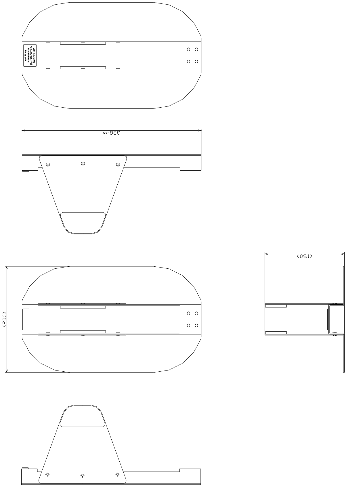
图 4-1 HC-TOKT-A01 外觀图
