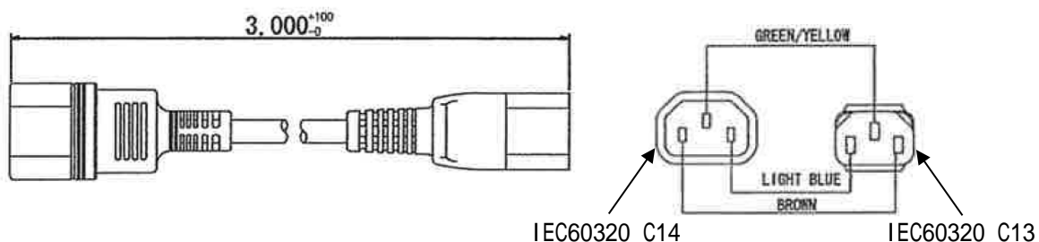
図 5-1 電源コードの外観図
