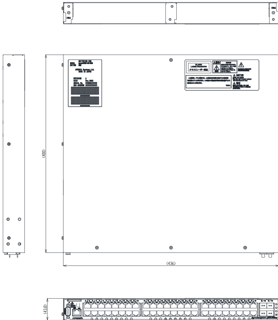
図 10-1 Apresia13200-48X-PSR3 外観図
