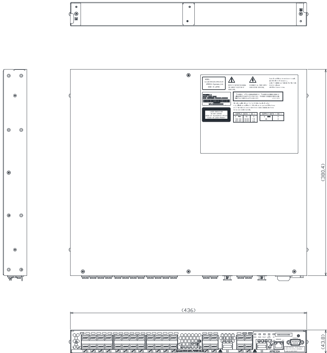
図 10-1 Apresia15000-32XL-PSR2-1GLIM 外観図
