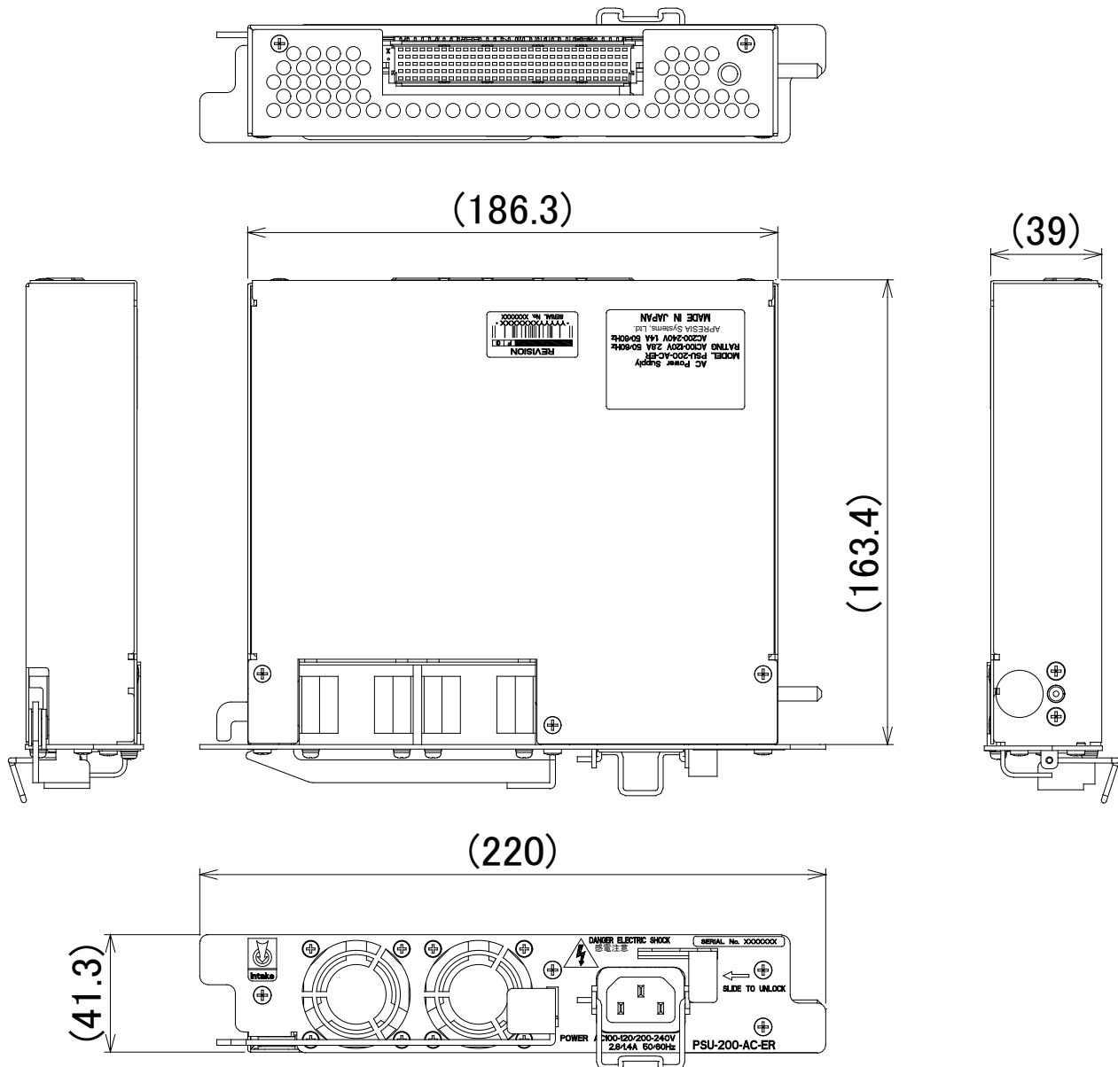
図 9-1 PSU-200-AC-ER 外観図
