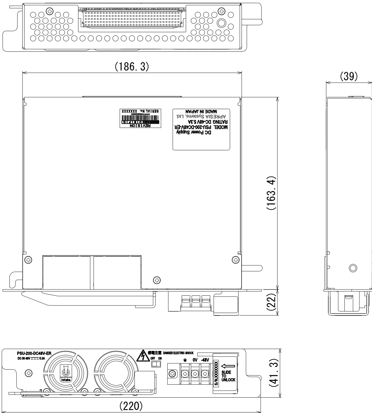
図 9-1 PSU-200-DC48V-ER 外観図
