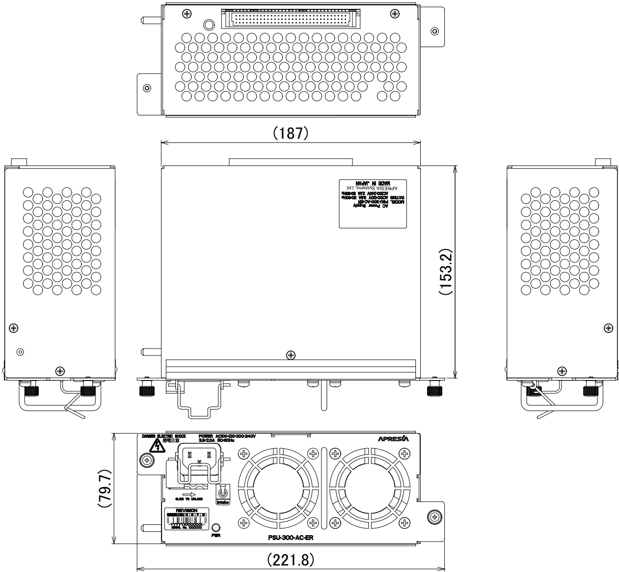
図 9-1 PSU-300-AC-ER 外観図
